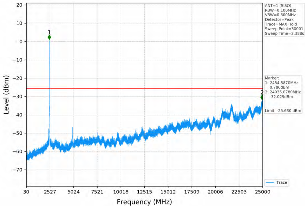
802.11n(HT20)_SISO_ANT1_REF
