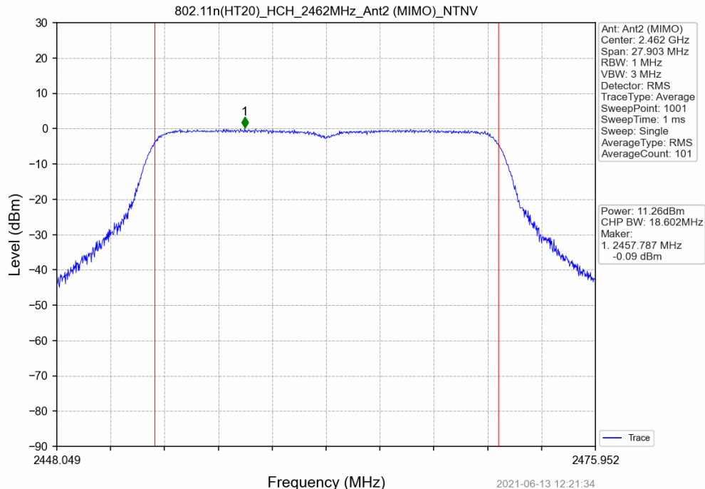
802.11n(HT20)_HCH_2462MHz_Ant2 (MIMO)_NTNV
