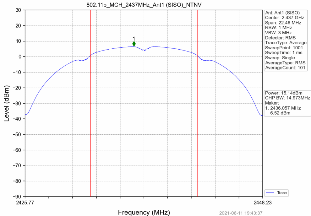
802.11b_MCH_2437MHz_Ant1 (SISO)_NTNV
