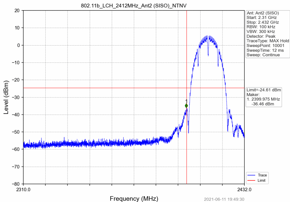
802.11b_LCH_2412MHz_Ant2 (SISO)_NTNV
