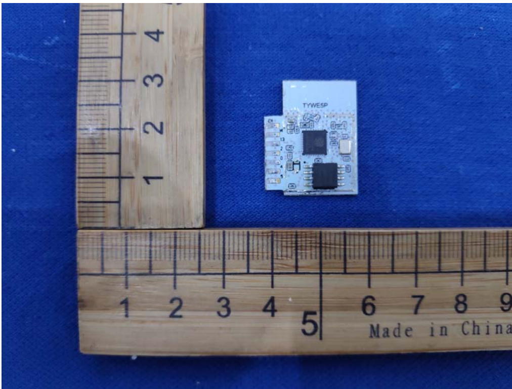
10) EUT Photo
