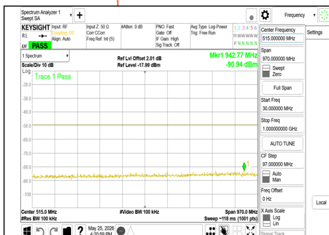
LPI 802.11be 160MHz Chain1 6185MHz Range1
