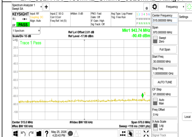
LPI 802.11be 160MHz Chain0 6185MHz Range1
