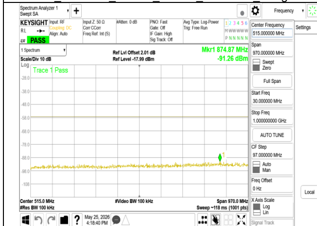
LPI 802.11be 160MHz Chain0 6025MHz Range1
