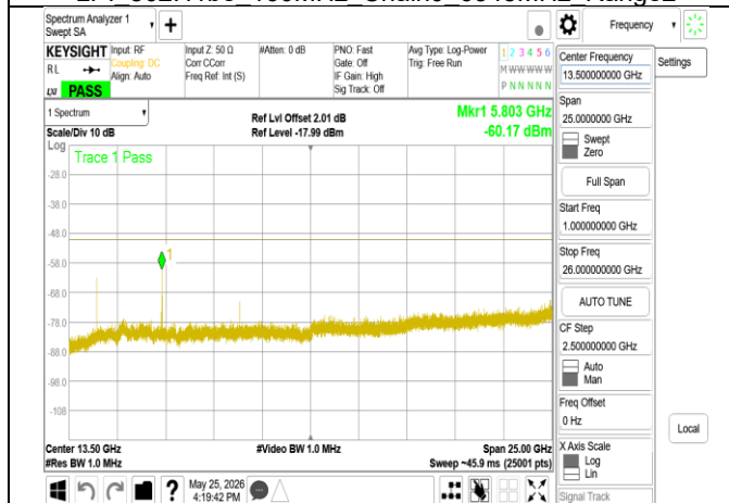
LPI_802.11be_160MHz_Chain1_6025MHz_Range2
