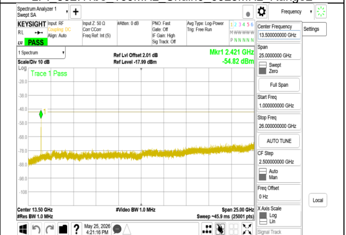
LPI 802.11be 160MHz Chain0 6185MHz Range2
