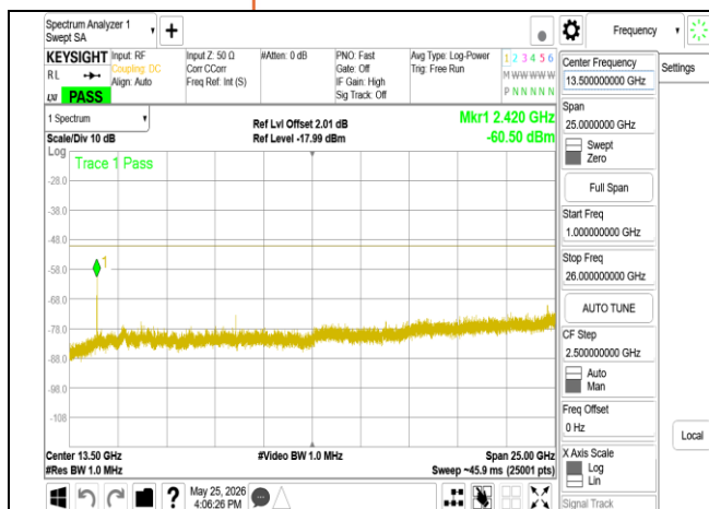
LPI 802.11be 80MHz Chain1 5985MHz Range2
