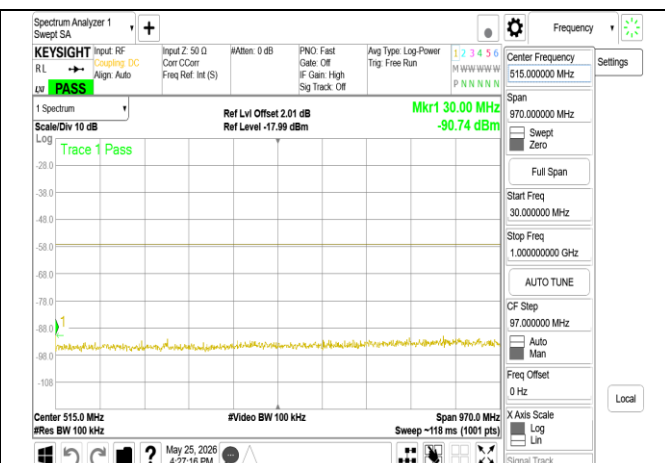
LPI_802.11be_320MHz_Chain1_6265MHz_Range1
