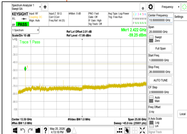
LPI 802.11be 80MHz Chain1 6385MHz Range2
