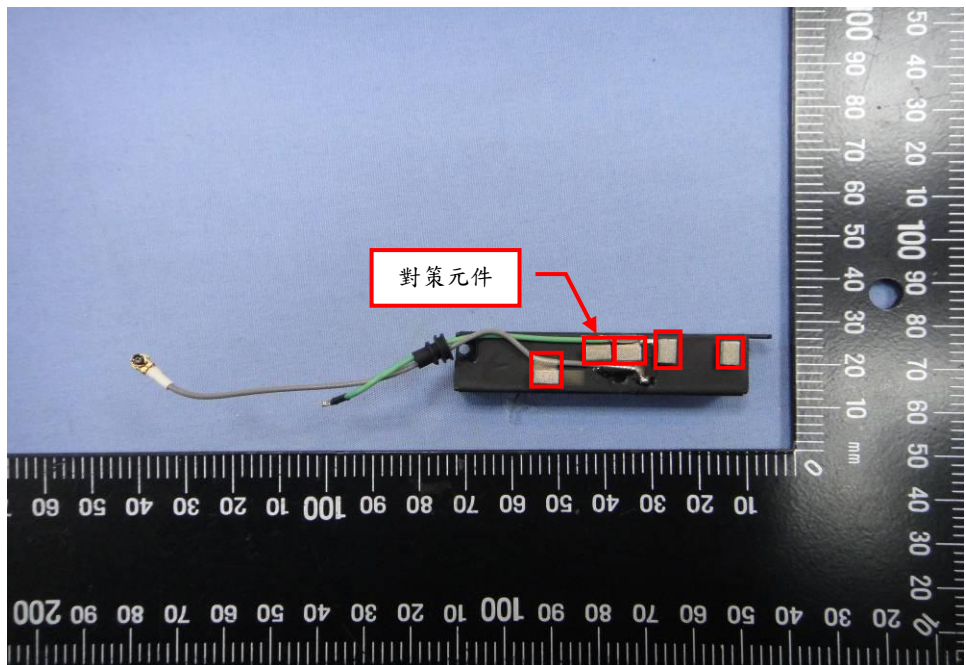
EUT Photo (16)
