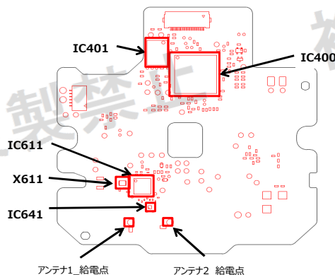
裏面部品配置
