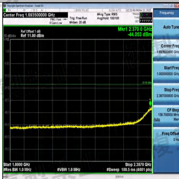
NTNV-11B-Ant1-2472-1000~2387-PASS
