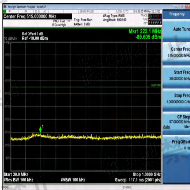
NTNV-11G-Ant1-2412-30~1000-PASS
