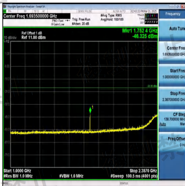
NTNV-11G-Ant1-2472-1000~2387-PASS
