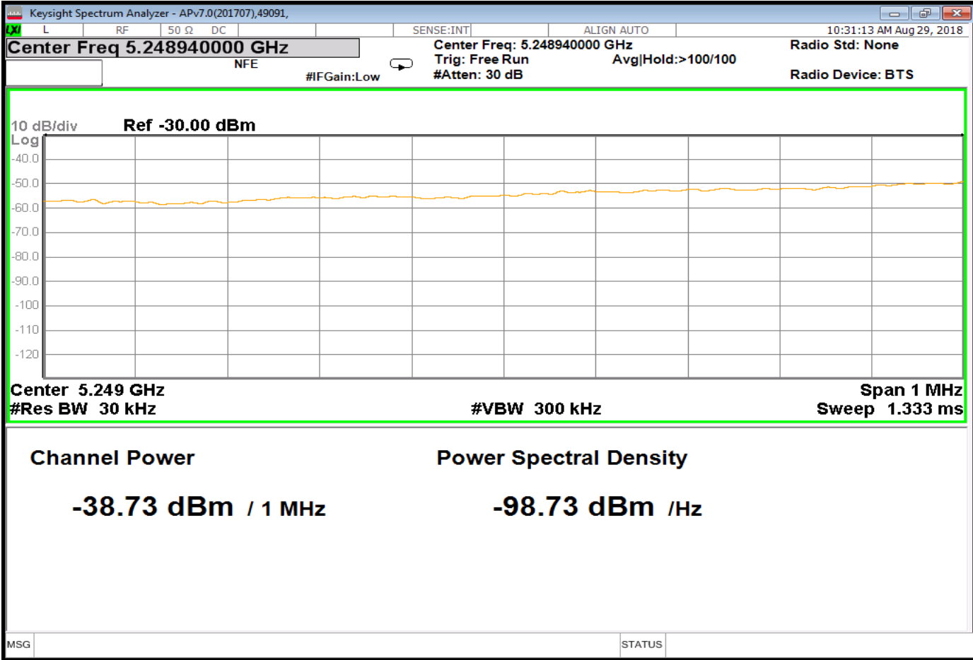
Tx1_Leak3Zoom_Nom
