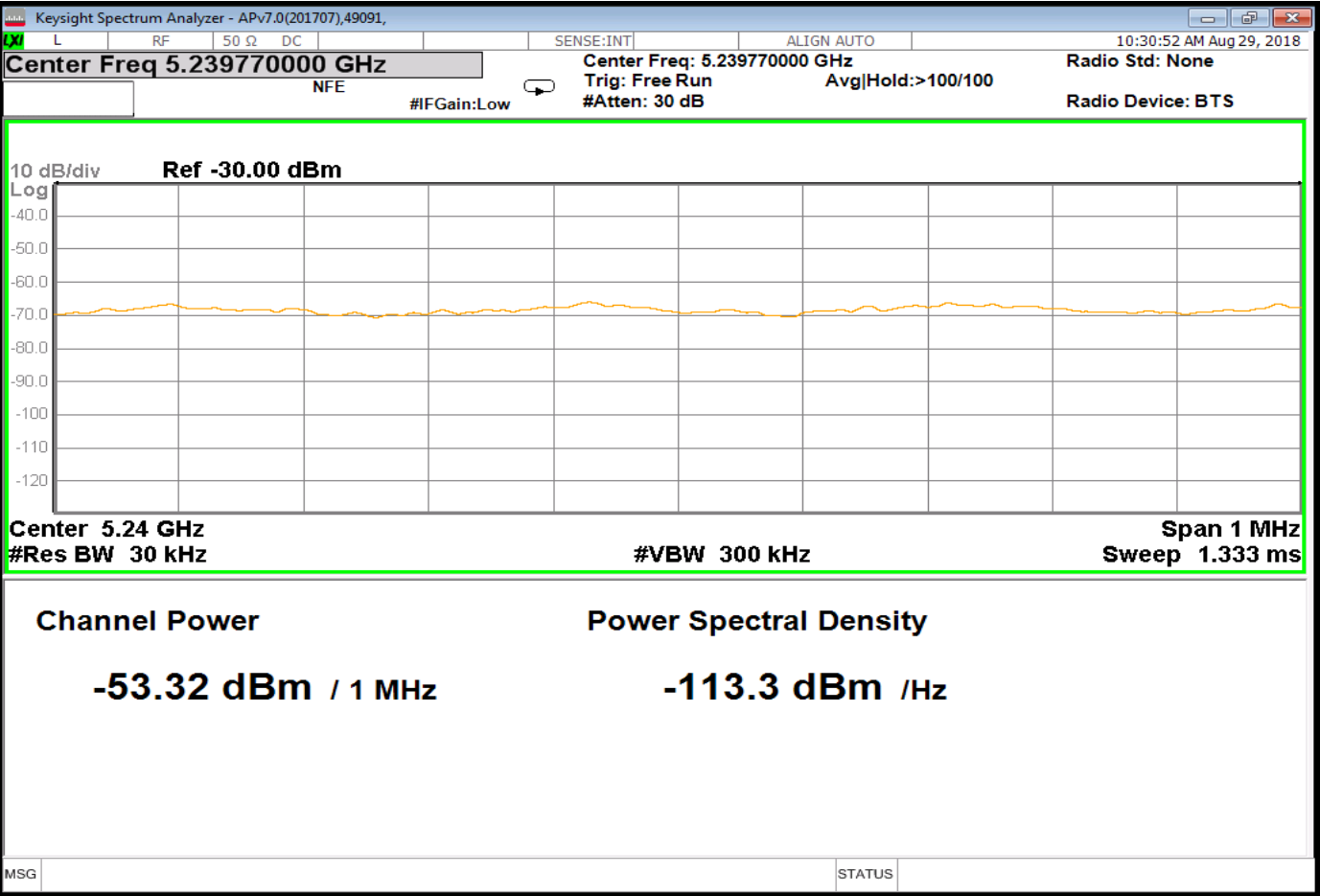
Tx1_Leak2Zoom_Nom
