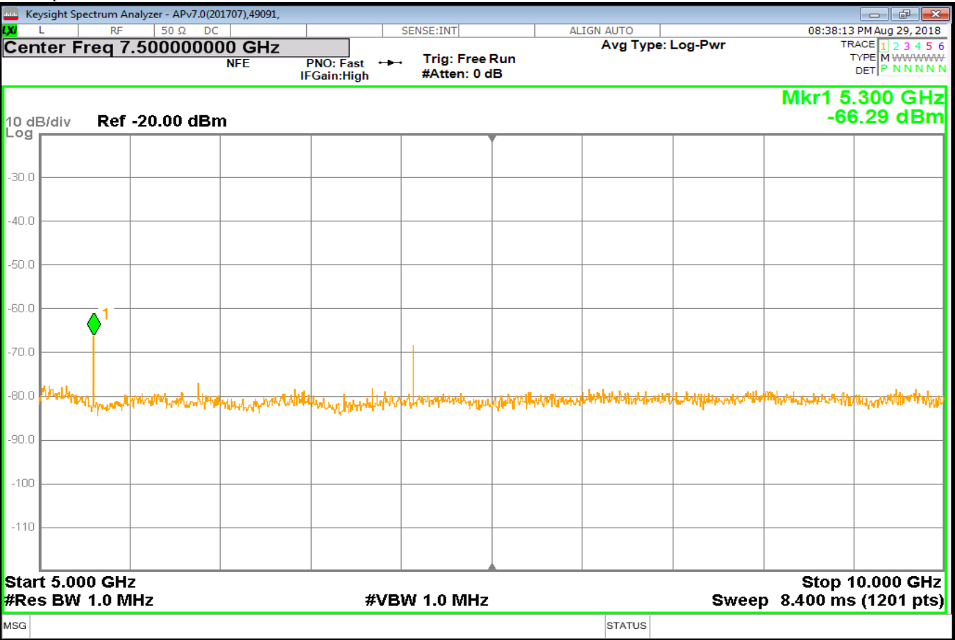
Rx1_SpuriousG2_Nom
