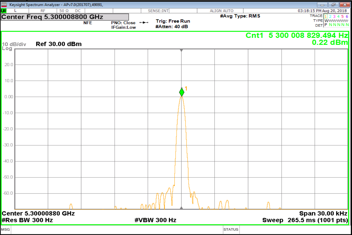
Tx2_Freq_Nom
