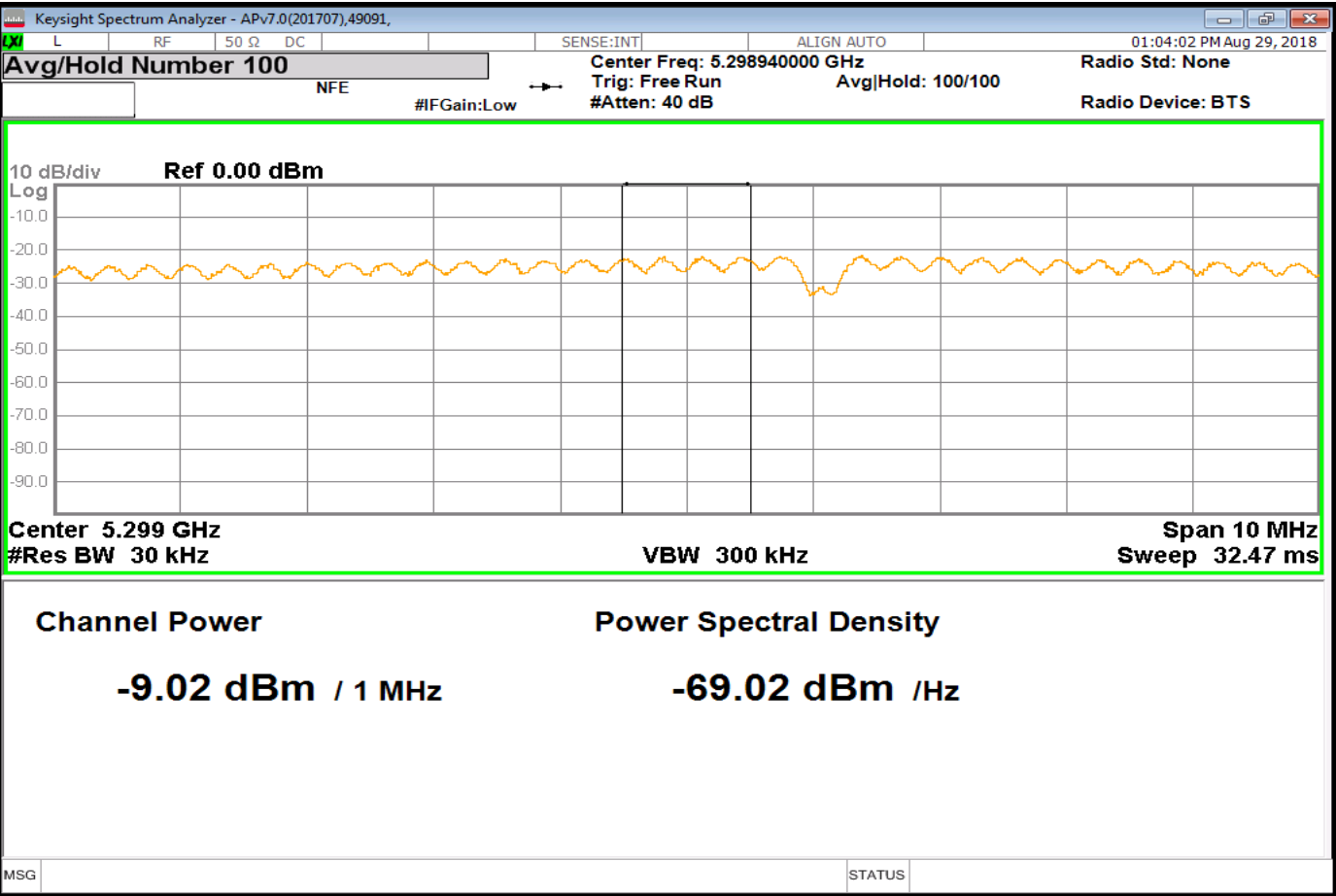
Tx2_Power_Chain0_Nom
