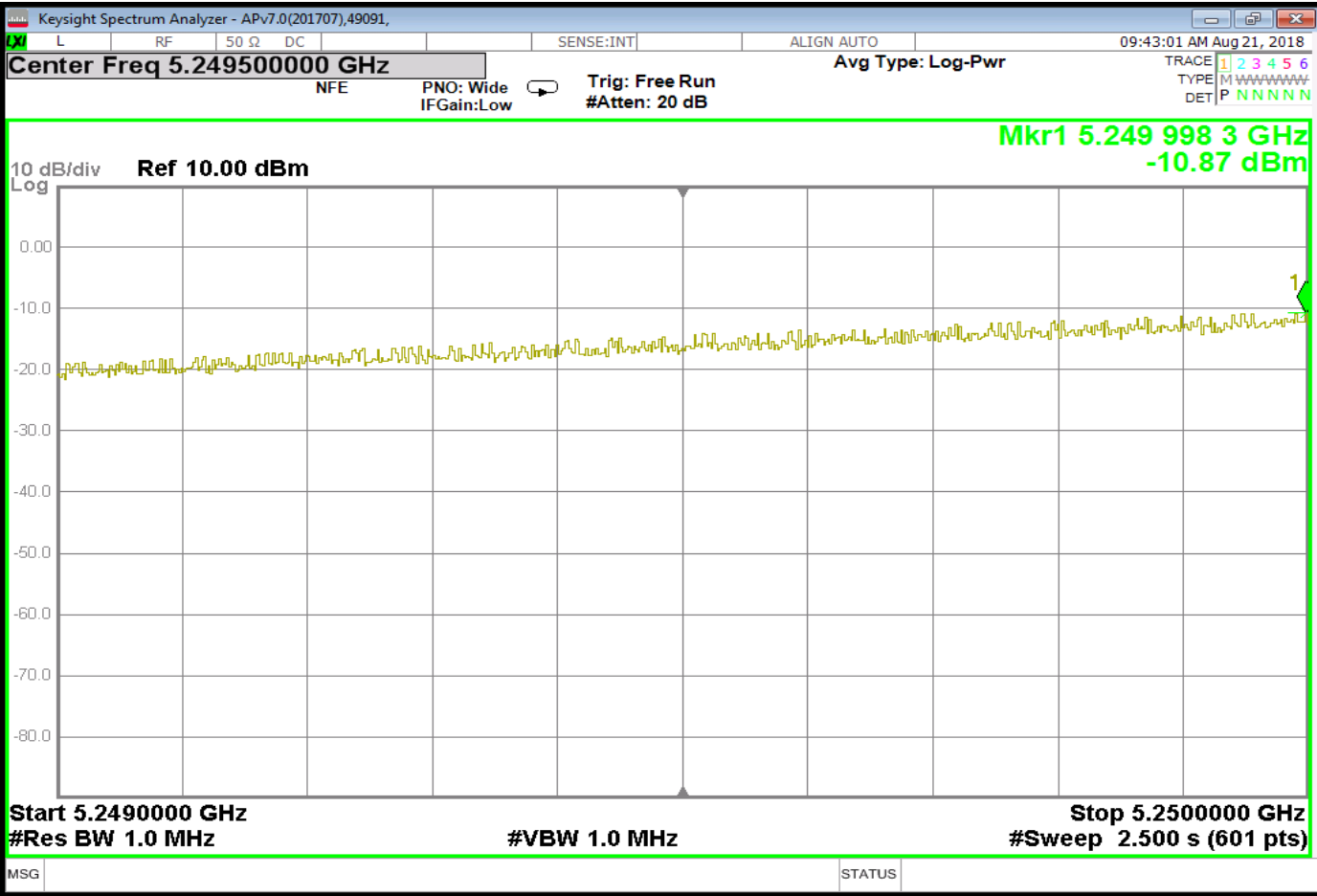
Tx1_Leak4_Nom
