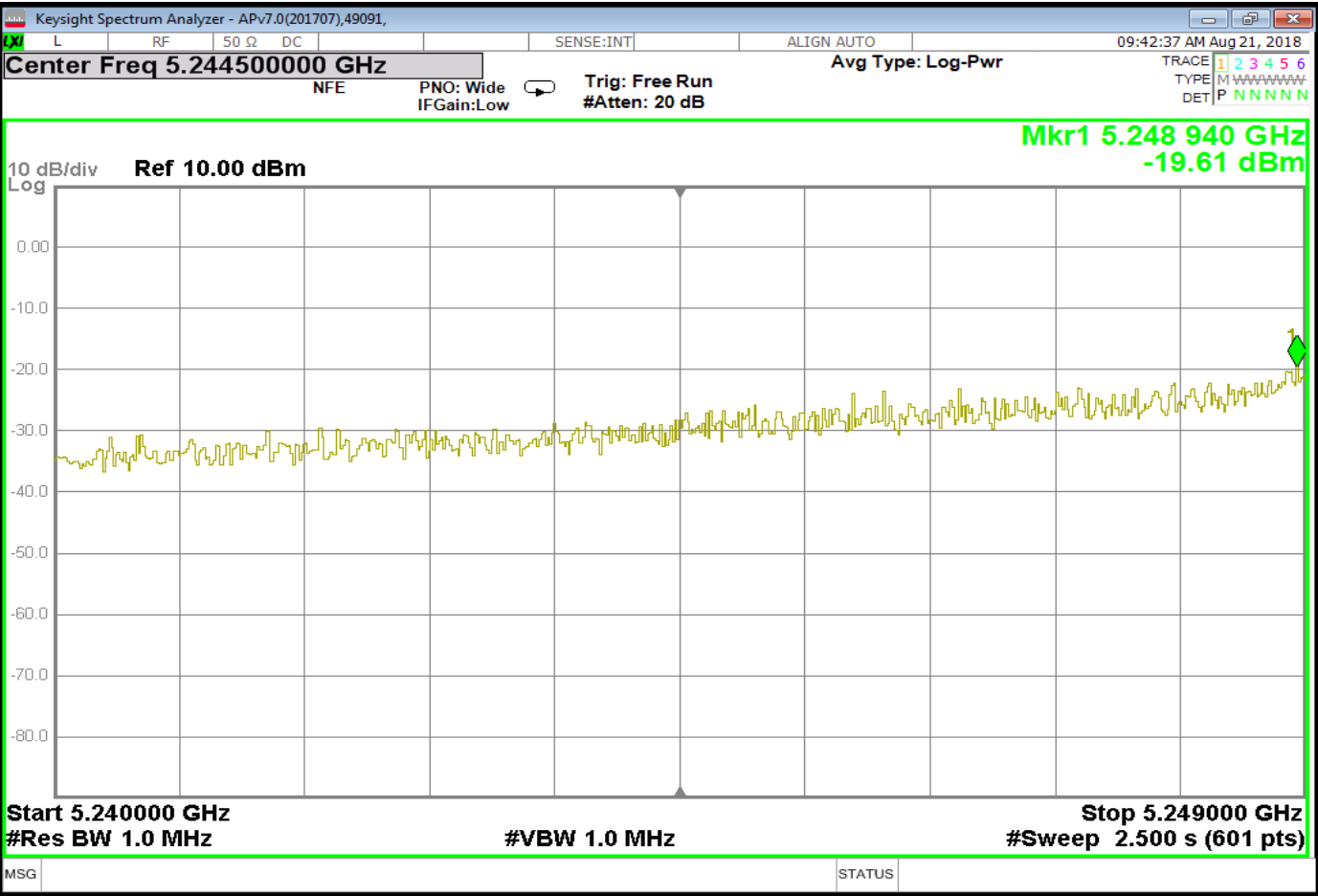
Tx1_Leak3_Nom
