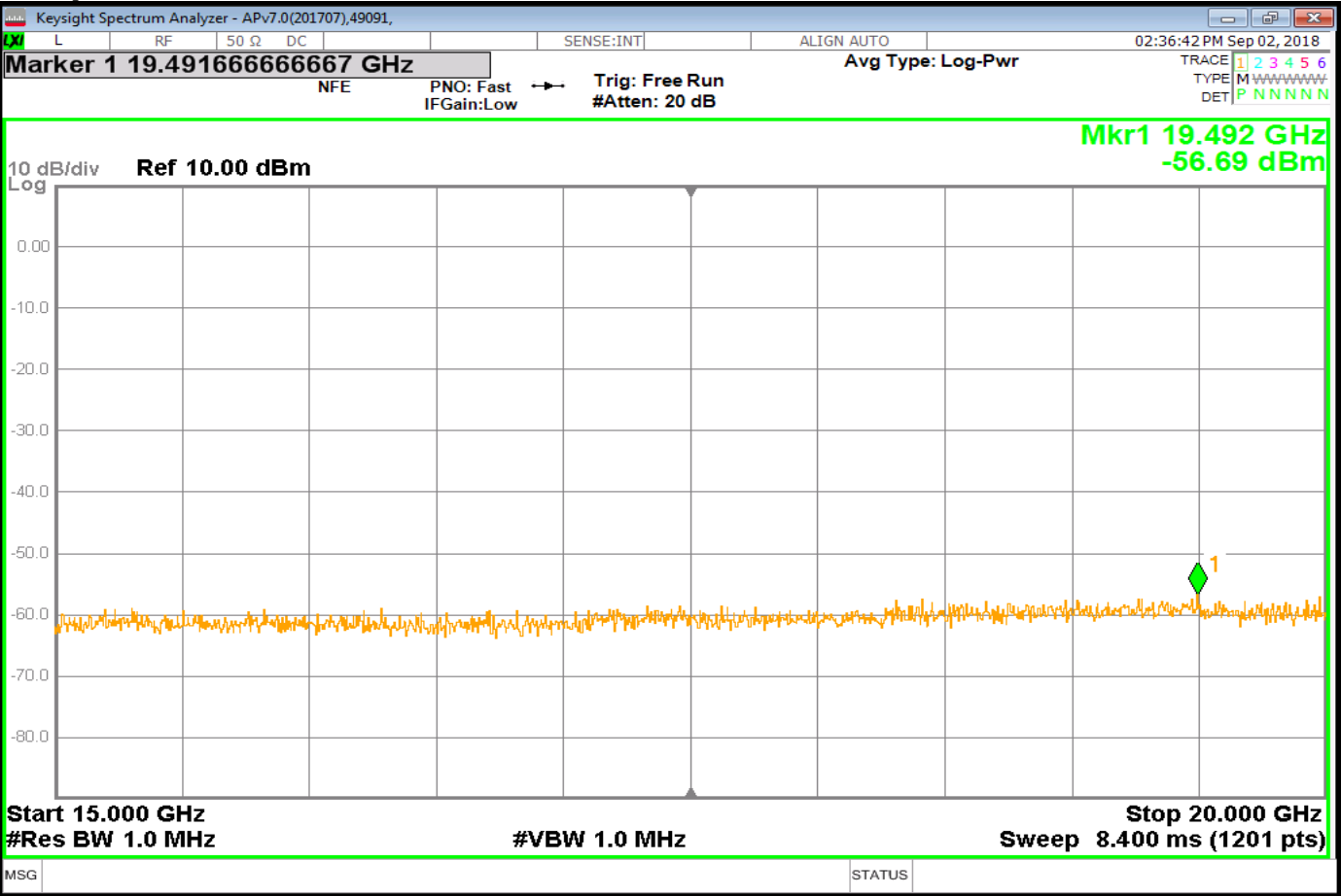
Tx2_SpuriousG4_Nom
