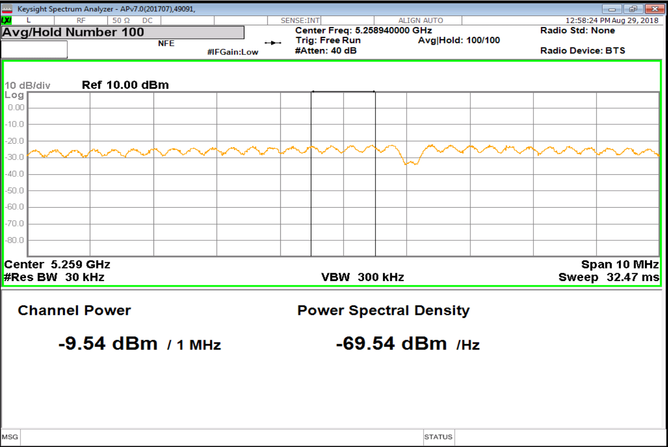
Tx1_Power_Chain0_Nom
