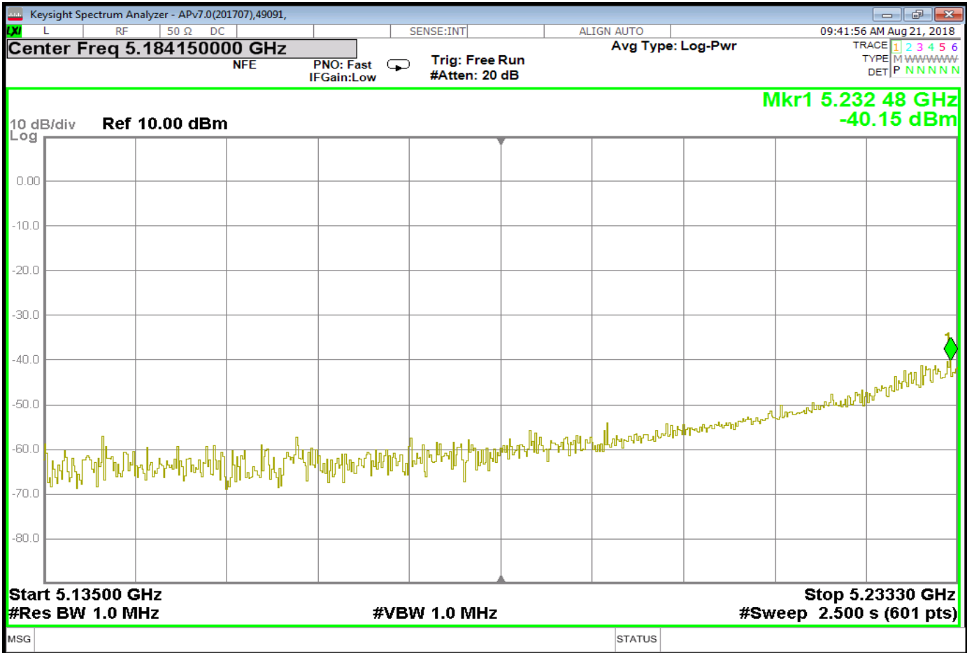
Tx1_Leak1_Nom
