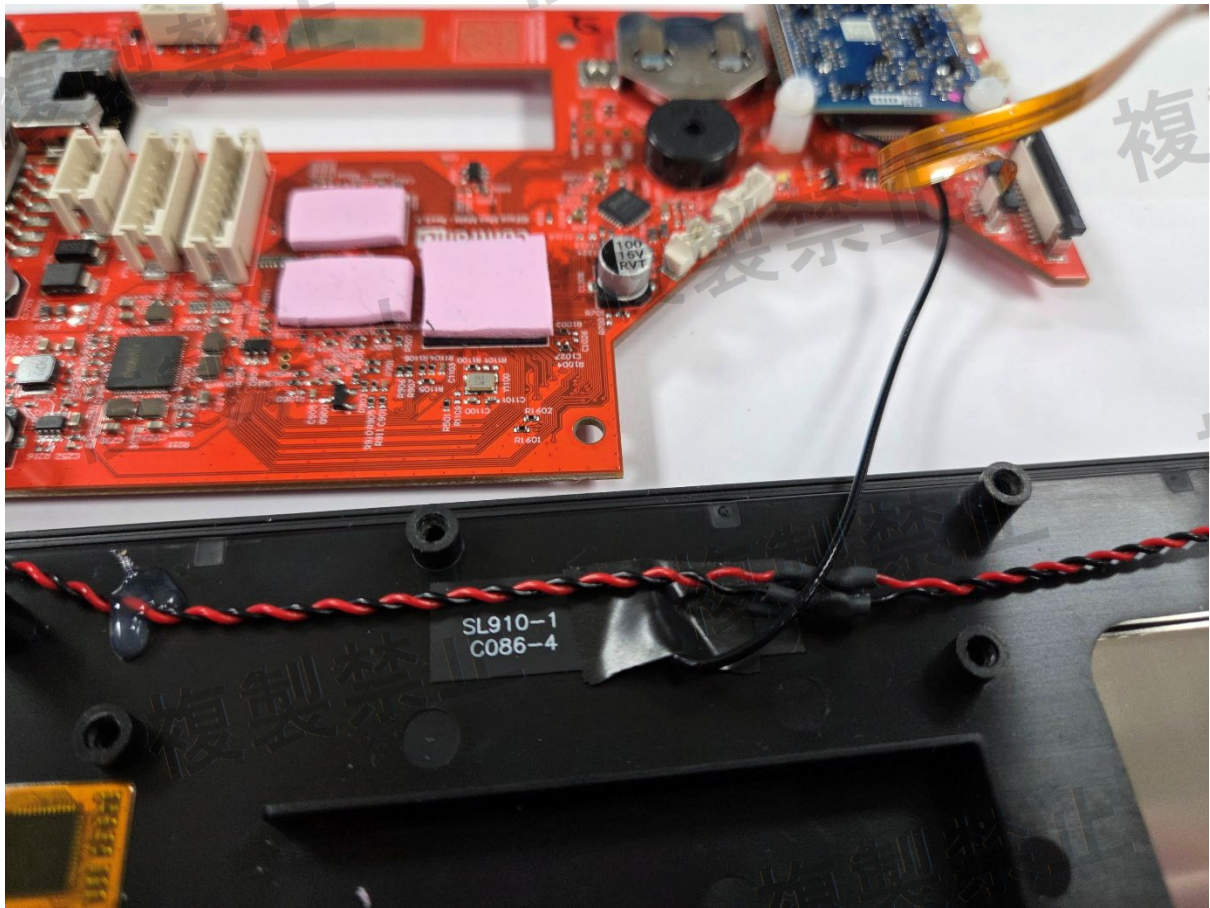
BLE Antenna position
