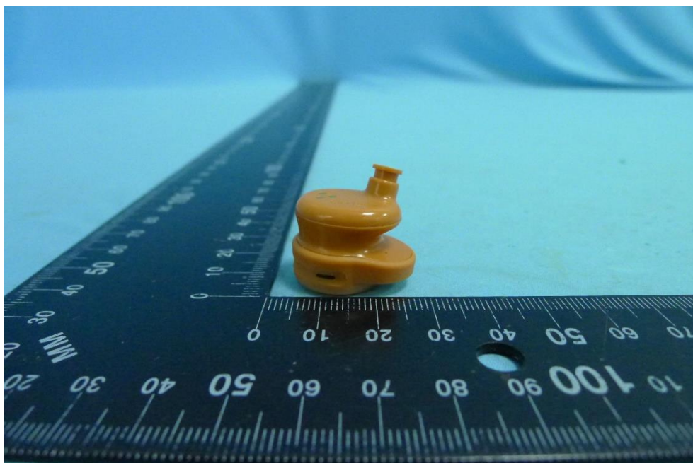
(3) 待測物照片 (左耳)
