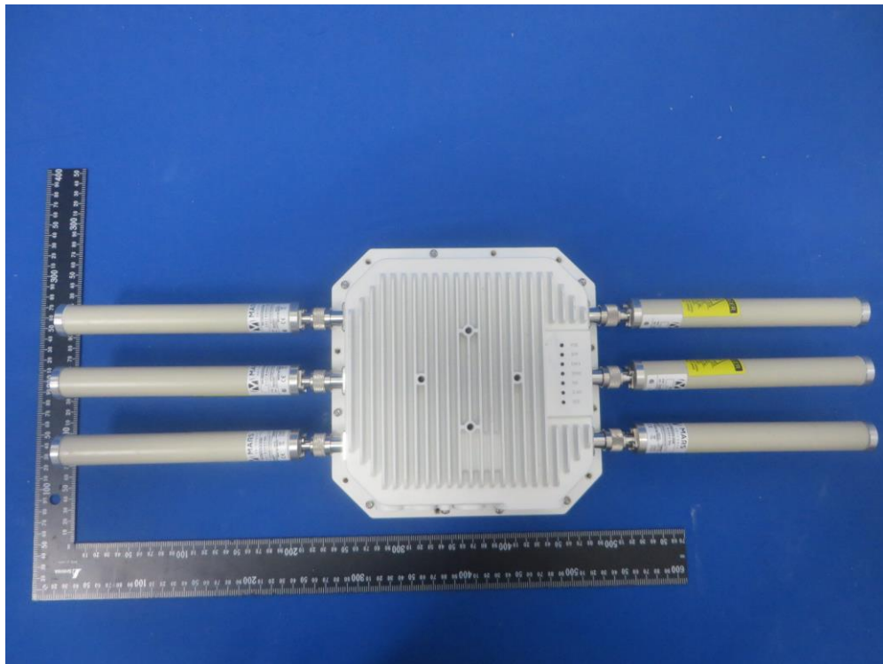
(15) EUT Photo - OAW-AP1362
