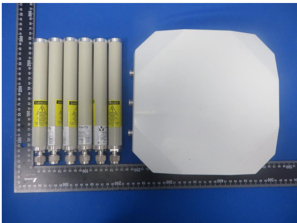
(16) EUT Photo - OAW-AP1362
