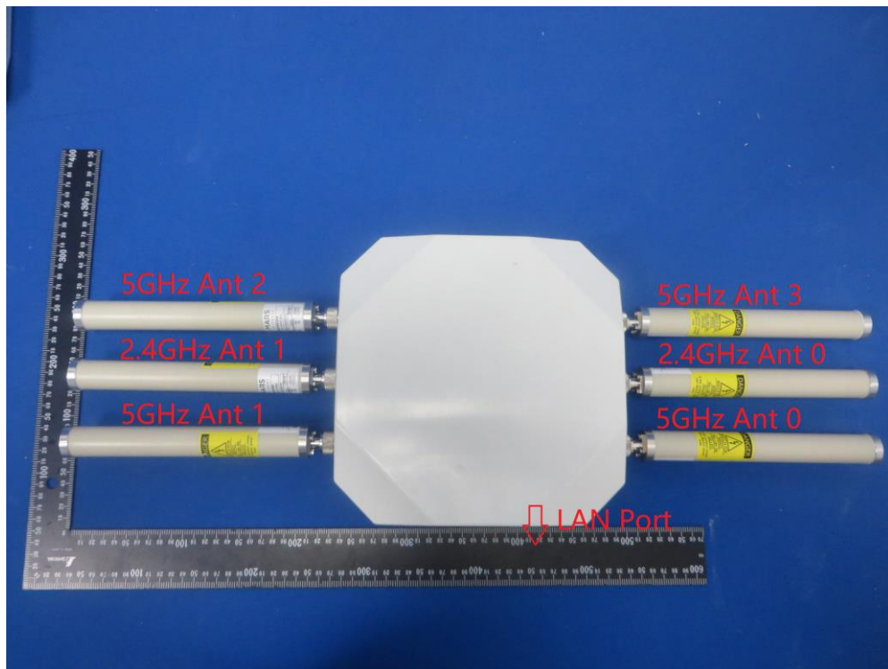
(13) EUT Photo - OAW-AP1362
