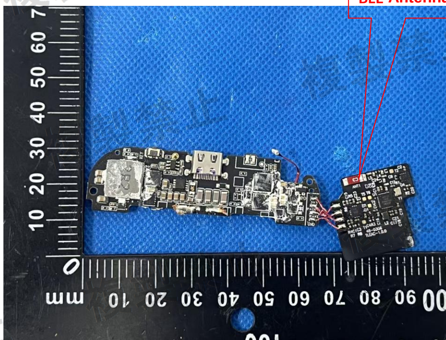
BLE Antenna
