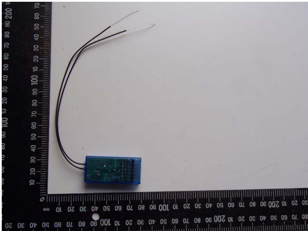
圖 18、設備 RX 側面照(廠牌: SANWA /型號: TX:AQUILA 6-4WD ; RX:RX-71E)
