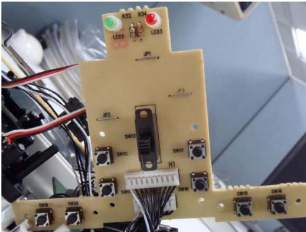
圖 6、TX-1 電路板零件面(廠牌: SANWA /型號: TX:AQUILA 6-4WD ; RX:RX-71E)
