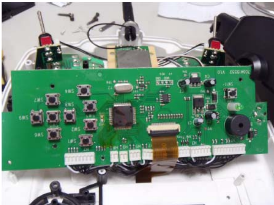
圖 12、TX-4 印刷電路板零件面(廠牌: SANWA /型號: TX:AQUILA 6-4WD ; RX:RX-71E)
