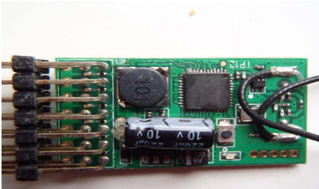
圖 20、設備 RX 印刷電路板零件面(廠牌: SANWA /型號: TX:AQUILA 6-4WD ; RX:RX-71E)
