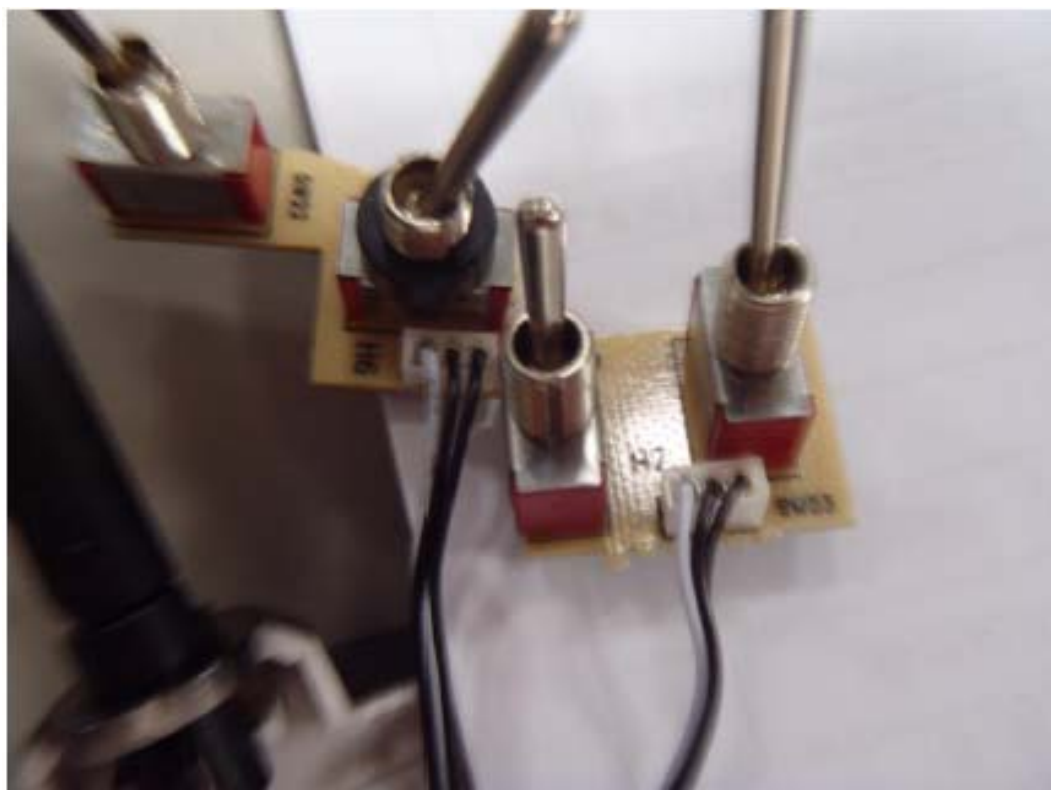
圖 8、TX-2 印刷電路板零件面(廠牌: SANWA /型號: TX:AQUILA 6-4WD ; RX:RX-71E)
