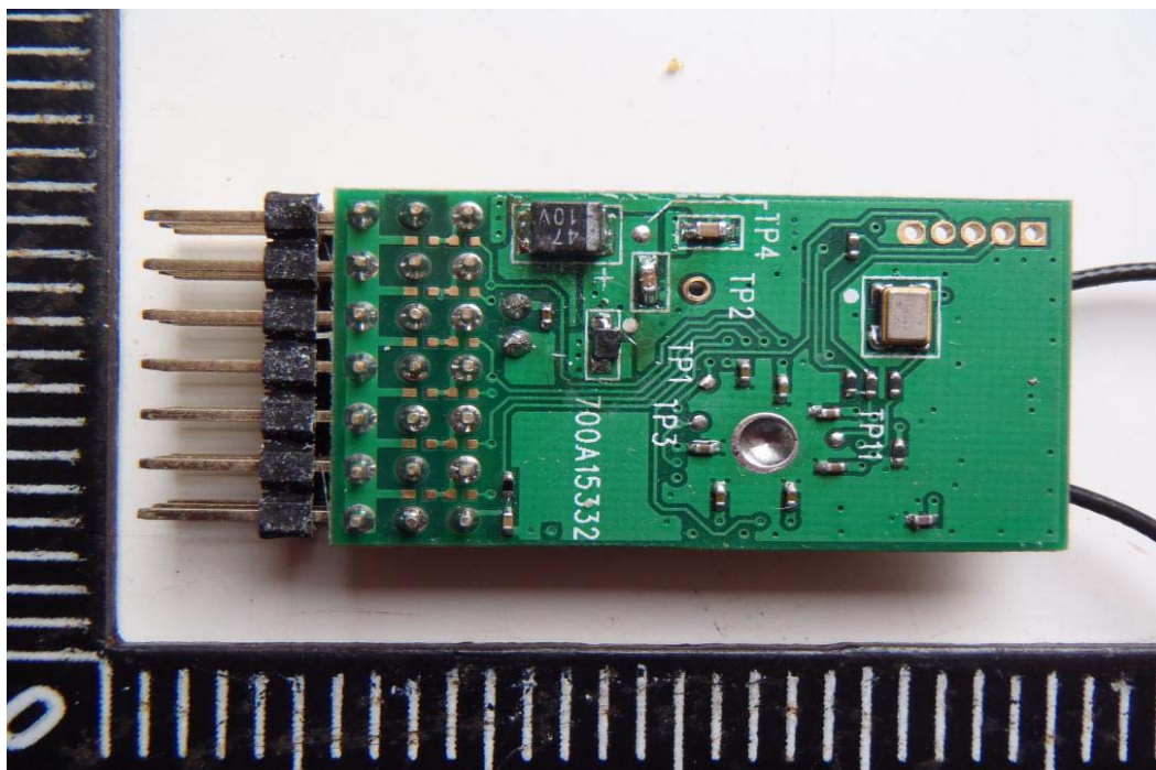
圖 21、設備 RX 印刷電路板銅軌面(廠牌: SANWA /型號: TX:AQUILA 6-4WD ; RX:RX-71E)
