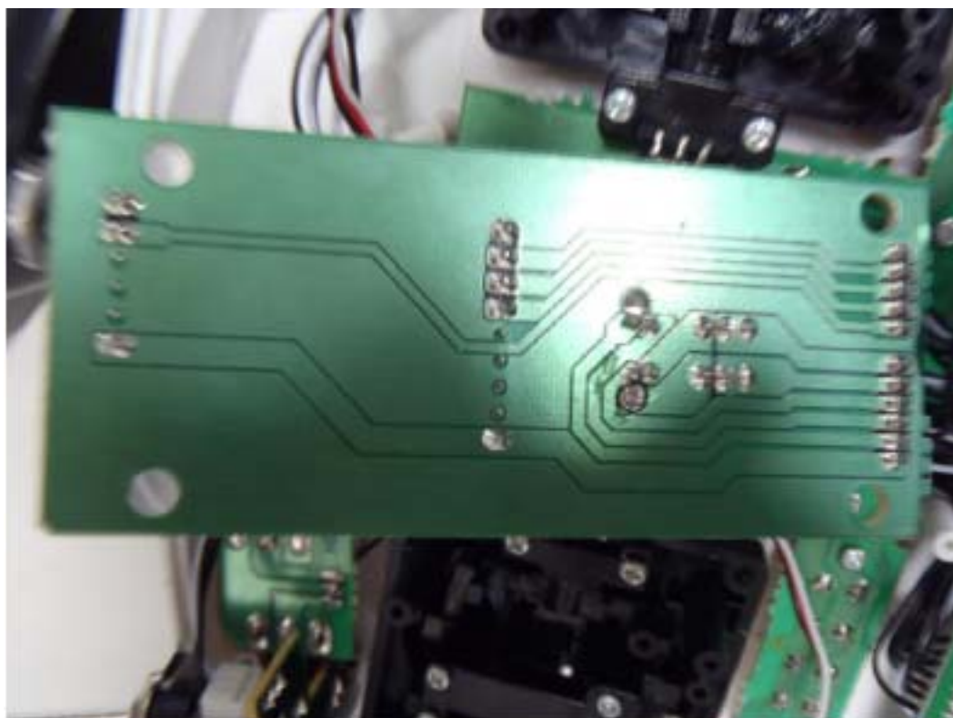
圖 16、設備 RX 正面照(廠牌: SANWA /型號: TX:AQUILA 6-4WD ; RX:RX-71E)
