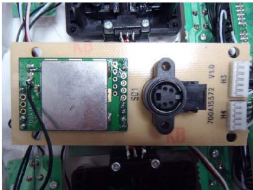
圖 14、TX-5 印刷電路板零件面(廠牌: SANWA /型號: TX:AQUILA 6-4WD ; RX:RX-71E)
