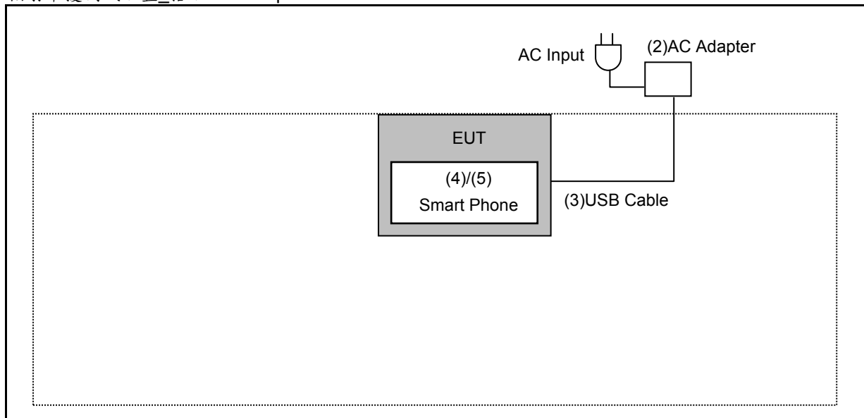
幅射干擾測試配置_搭配 AC Adapter
