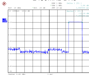
2480MHz-DH3
