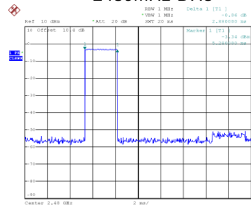
2480MHz-DH5
