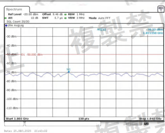
1805.0-1845.0_new Band 3 20MHz/1747.5/Mid QPSK 48@0
