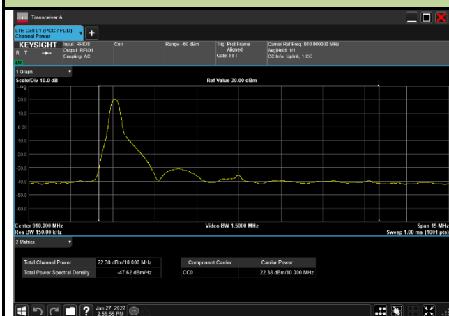
Band8 10MHz CH21750 1RB#0
