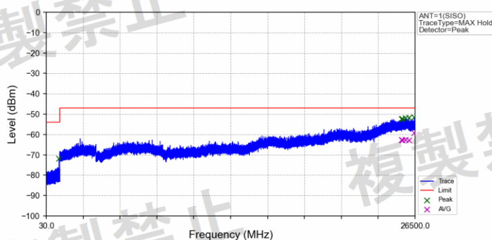
802.11ac(VHT20)_LCH_5500MHz_Ant1_NTNV
