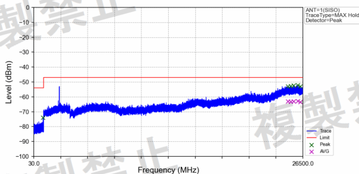
802.11ac(VHT80)_MCH_5210MHz_Ant1_NTNV
