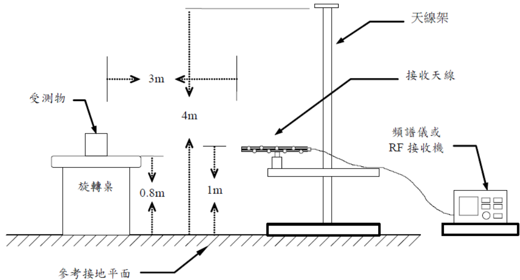
圖 1：量測頻率低於 1GHz 之測試配置
