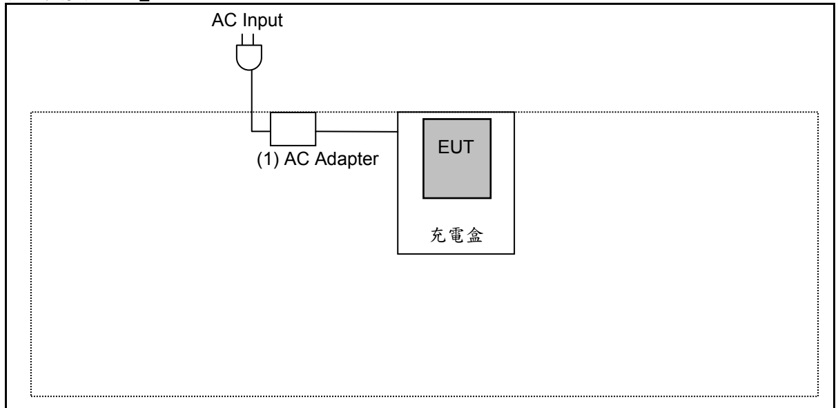
輻射干擾測試配置_30 MHz~1 GHz
