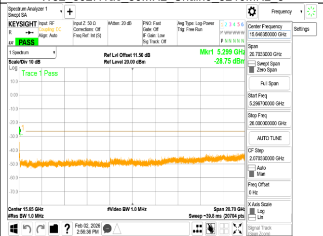
W52_802.11ac_80MHz_Chain0_5210MHz_6
