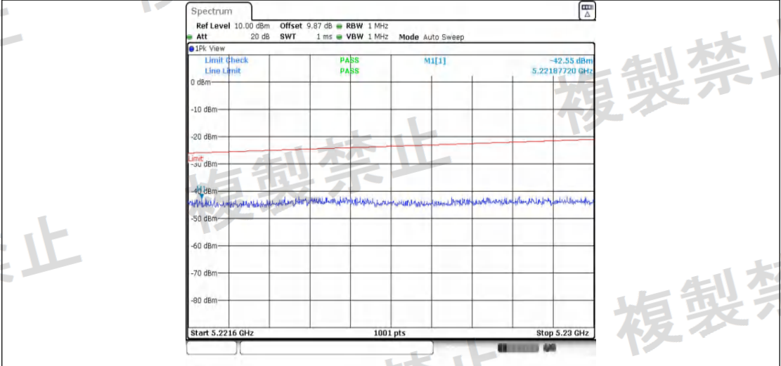
NTNV 11AX40MIMO Ant1 5270 5221.6~5230
