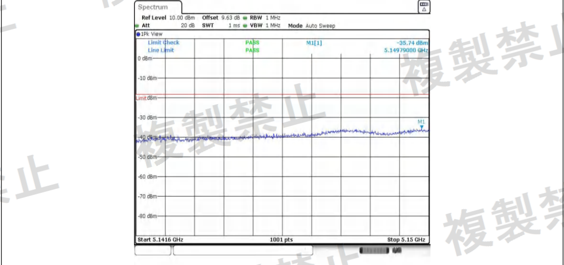
NTNV_11AX40MIMO_Ant2_5190_5141.6~5150
