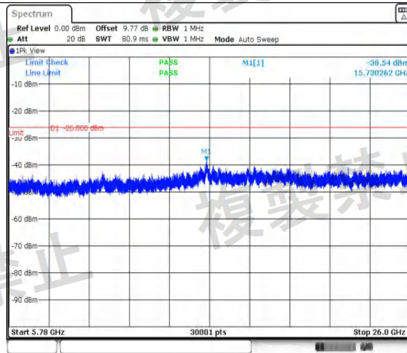
NTV 11AX20MIMO_Ant2 5500 5780~26000
