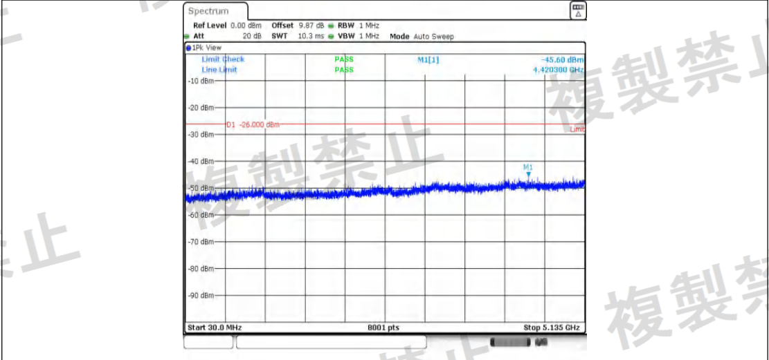
NTNV 11AX20MIMO_Ant1 5240 30~5135
