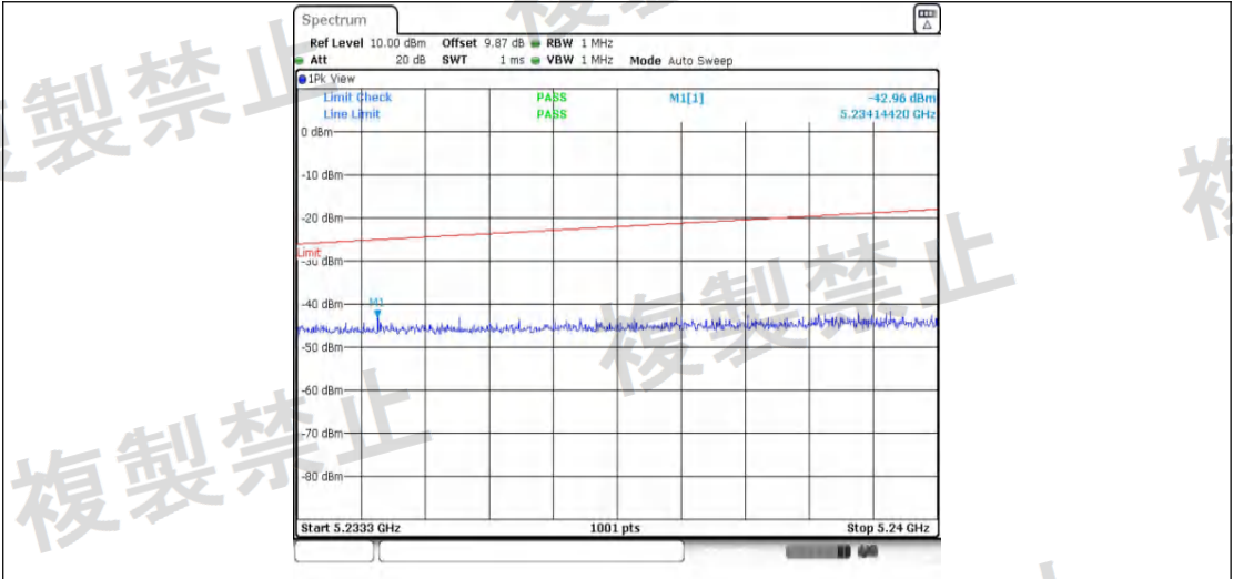
NTNV 11AX20MIMO Ant1 5260 5233.3~5240
