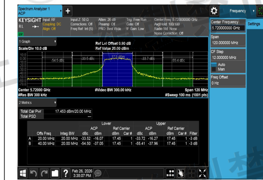
NTHV-11AC20SISO-Ant1-5720-PASS
