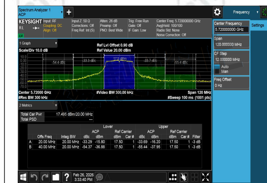
NTLV-11AC20SISO-Ant1-5720-PASS
