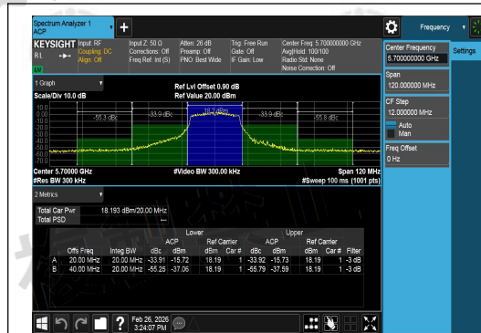
NTVN-11AC20SISO-Ant1-5700-PASS
