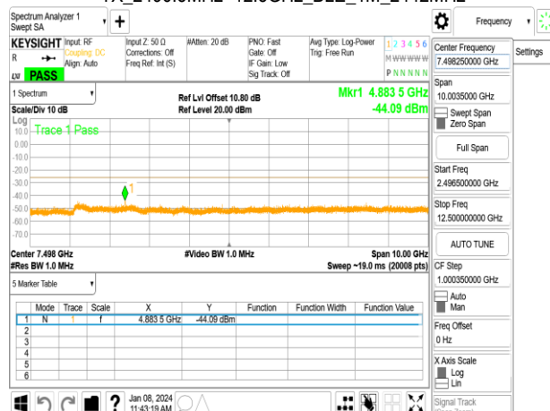
TX_2496.5MHz~12.5GHz_BLE_1M_2480MHz
