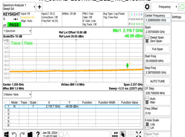
TX_30MHz~2387MHz_BLE_1M_2480MHz
