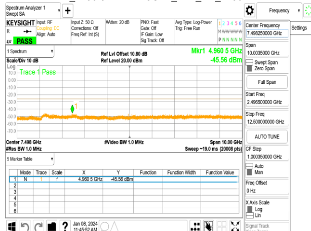
TX_2496.5MHz~12.5GHz_BLE_1M_2480MHz
