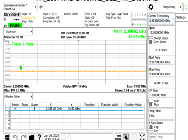
TX_2387MHz~2400MHz_BLE_1M_2480MHz
