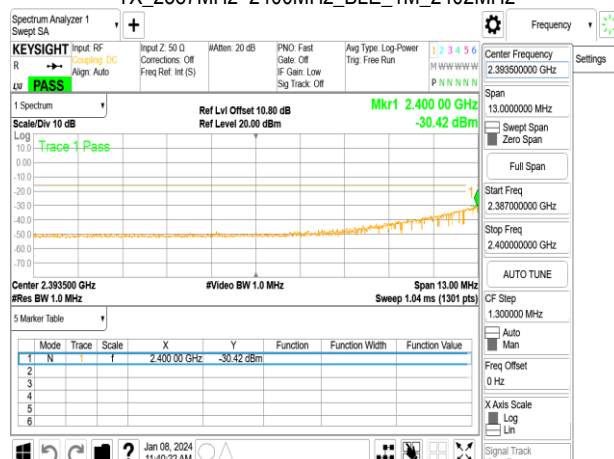
TX_2387MHz~2400MHz_BLE_1M_2442MHz
