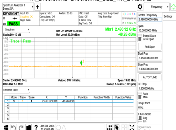
TX_2483.5MHz~2496.5MHz_BLE_1M_2480MHz
