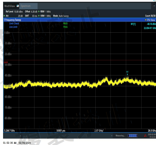
NTVN-11N20MIMO-Ant3-5200-5266.7~26000-P ASS
