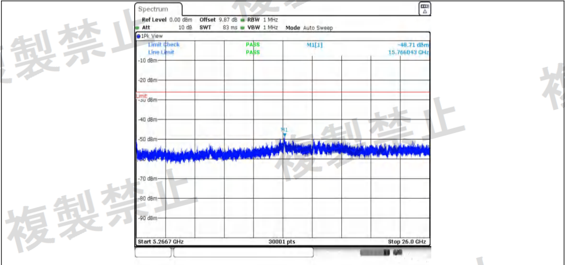
NTNV 11BE20MIMO_Ant1 5240_5266.7~26000
