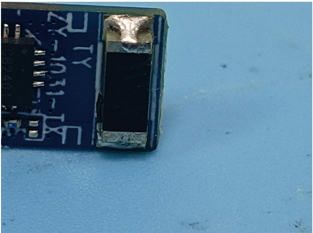
Antenna
