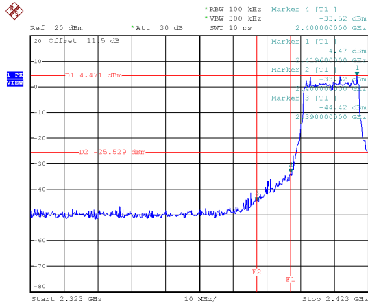
IEEE 802.11g 頻帶範圍外(下邊緣頻帶)之任意 100 kHz 內最大射頻功率
