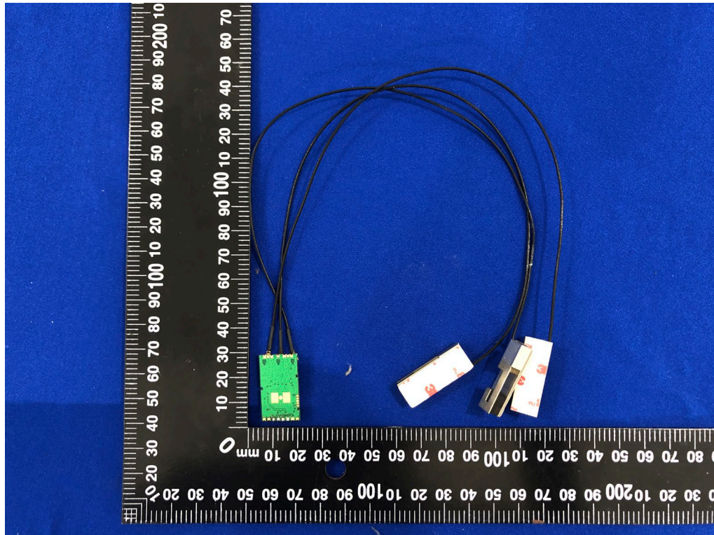
GSD / WIFI+BT Module / DCT2CM2101
