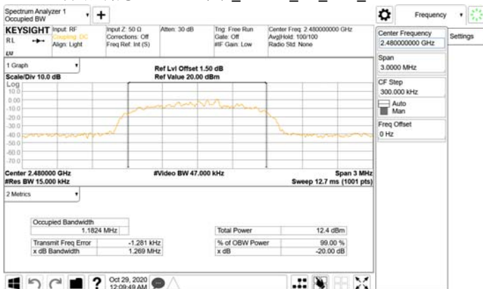
發射頻寬 20dB 之要求_8DPSK_3M_DH5_2480MHz
