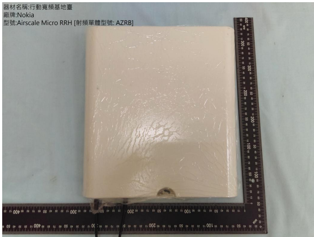
圖十. Antenna
