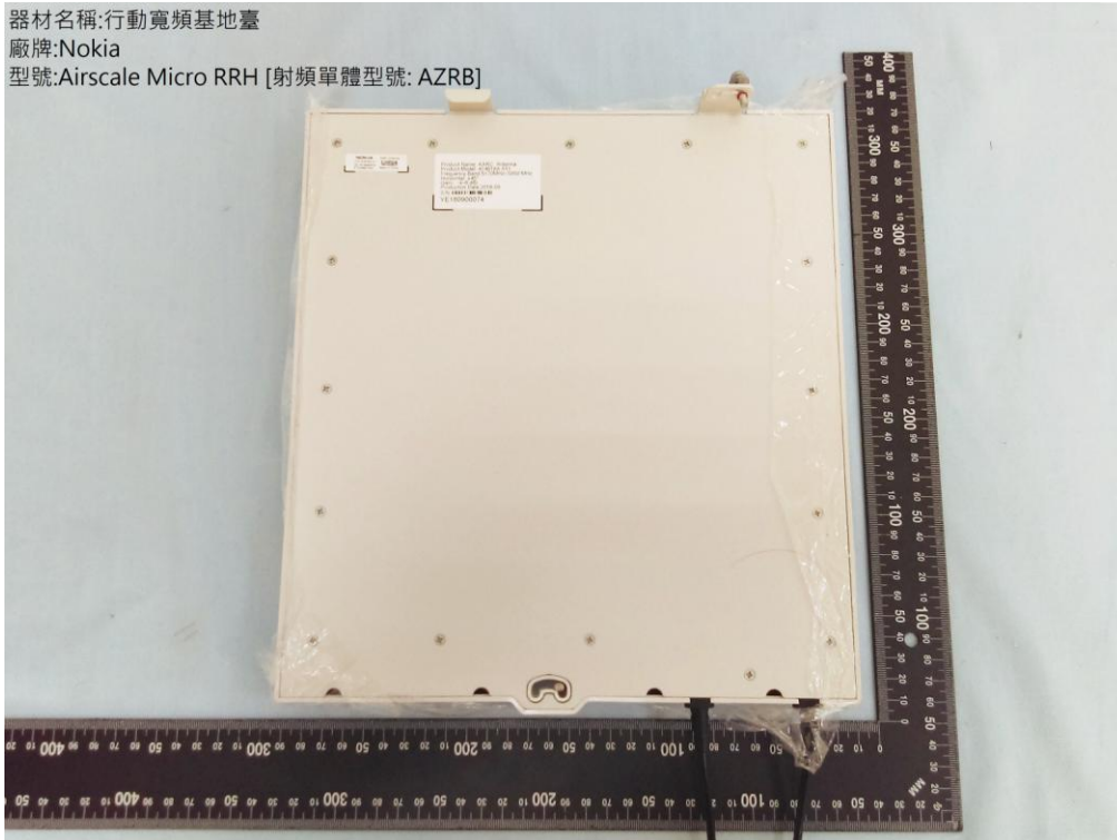
圖十一. 天線
