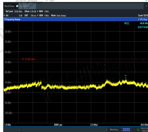
NTNV-11AC80SISO-Ant1-5690-1000~26000-PA SS
