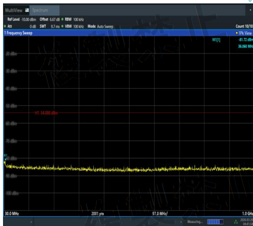
NTNV-11AX80SISO-Ant1-5610-30~1000-PASS
