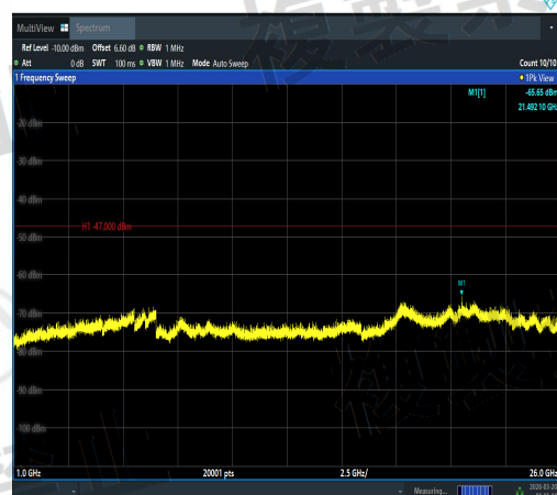
NTNV-11AX80SISO-Ant3-5530-1000~26000-PA SS
