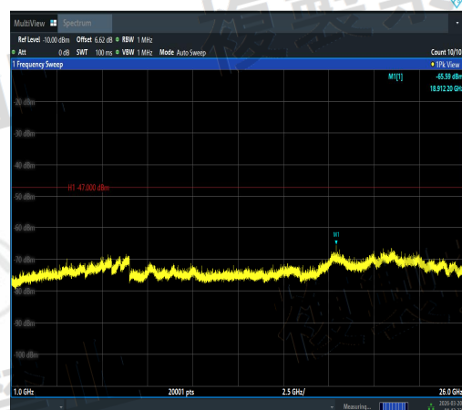
NTVN-11AX80SISO-Ant3-5690-1000~26000-PA SS
