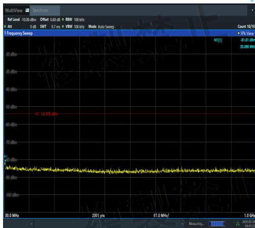
NTNV-11AX80SISO-Ant3-5530-30~1000-PASS
