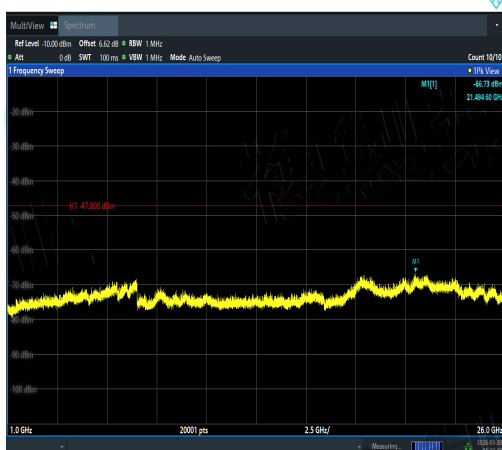
NTVN-11AX80SISO-Ant2-5690-1000~26000-PA SS
