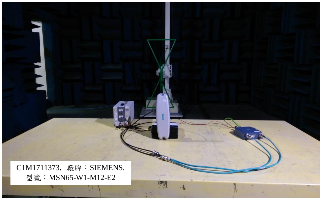
天線 No. 15: ANT795-6MT (站立)
