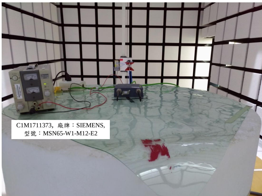
天線 No. 9: ANT795-4MC (側立)
