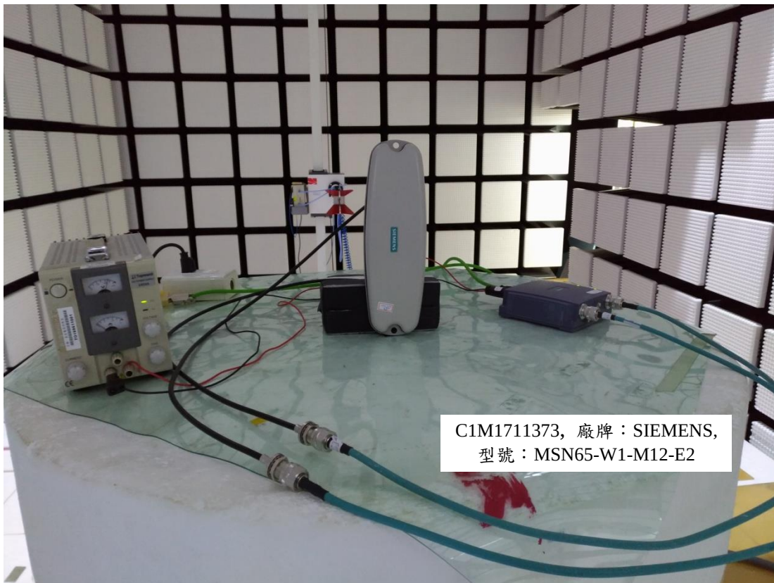
天線 No. 15: ANT795-6MT (站立)
