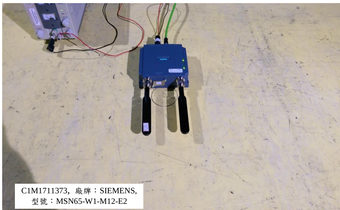
天線 No. 9: ANT795-4MC (平躺-Zoom View)
