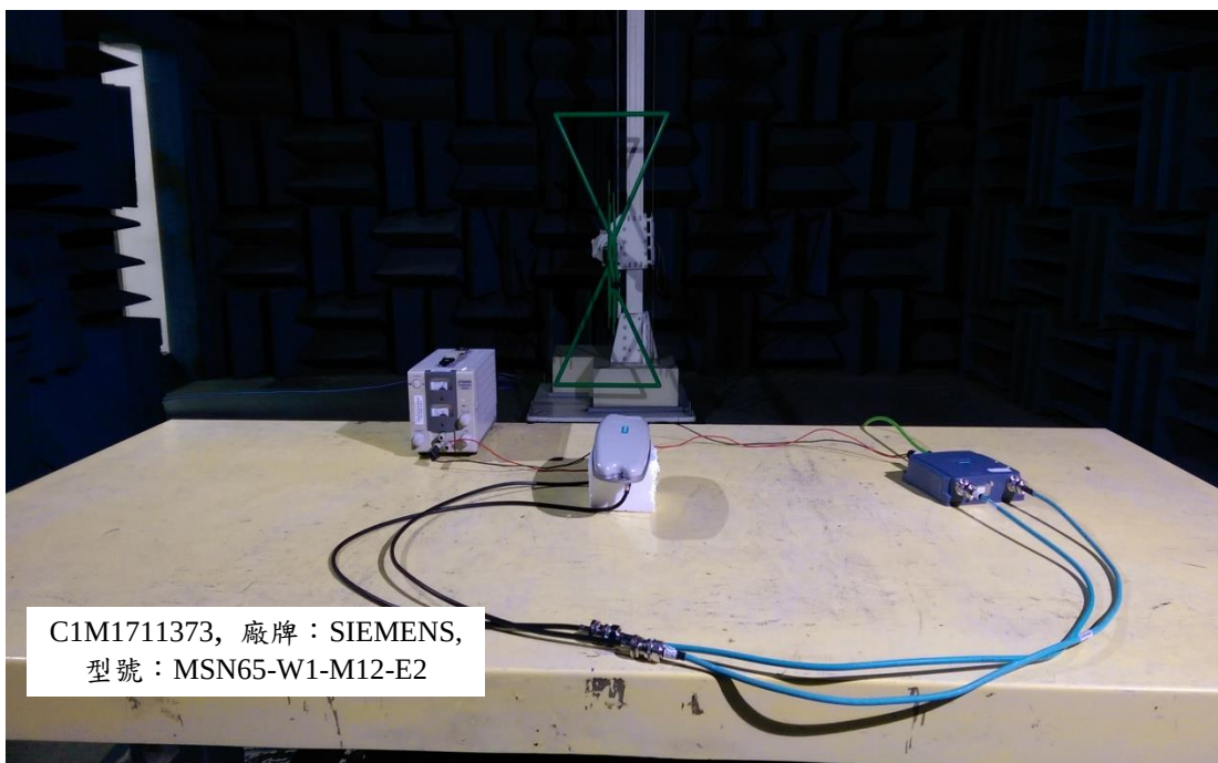
天線 No. 15: ANT795-6MT (平躺)
