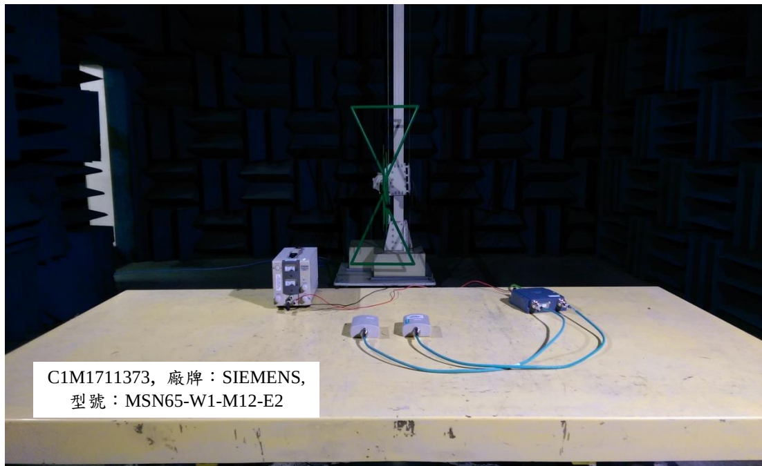
天線 No. 3: ANT795-6DC (平躺)
