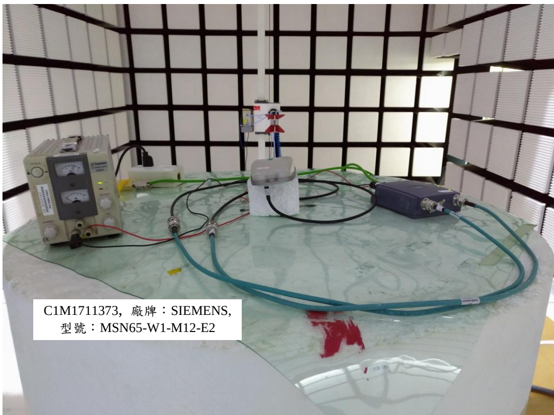
天線 No. 15: ANT795-6MT (平躺)
