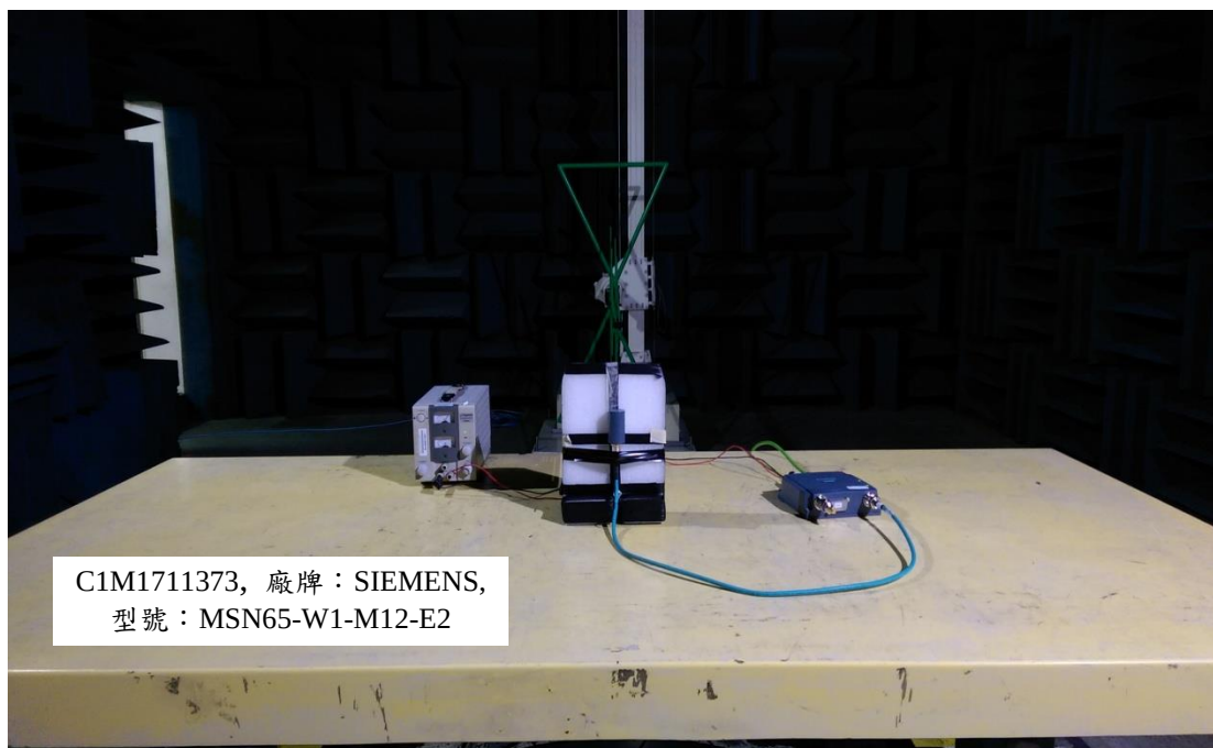
天線 No. 12: ANT793-4MN (站立)
