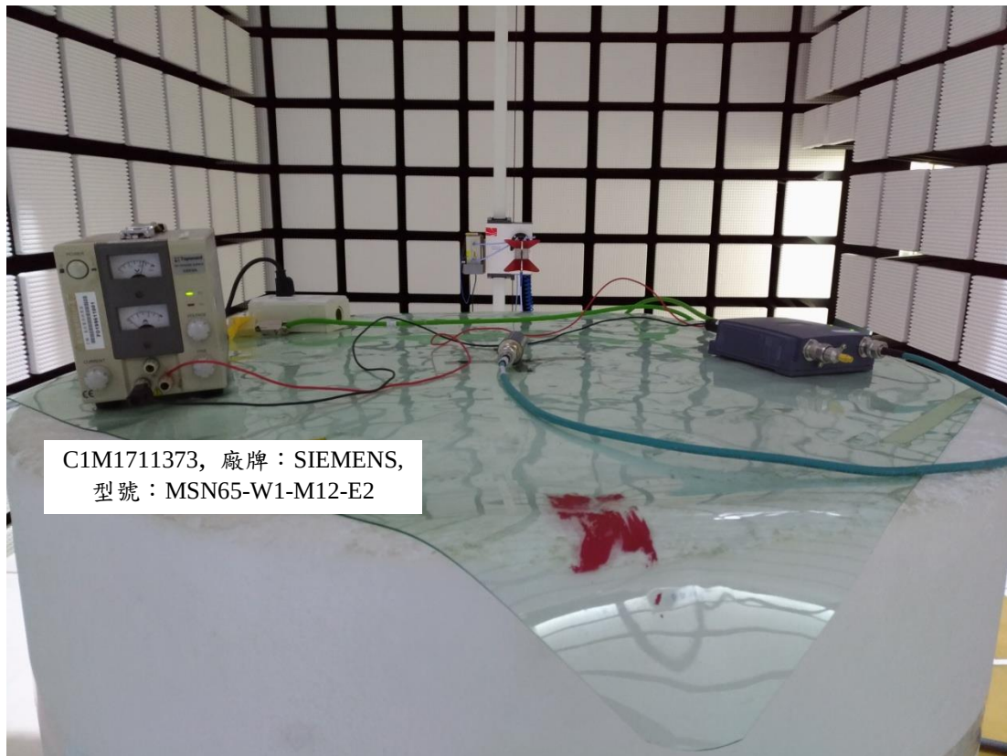
天線 No. 12: ANT793-4MN (平躺)
