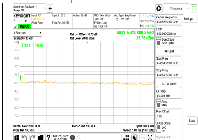
VLP 802.11ax 20MHz Chain1 6415MHz Range2
