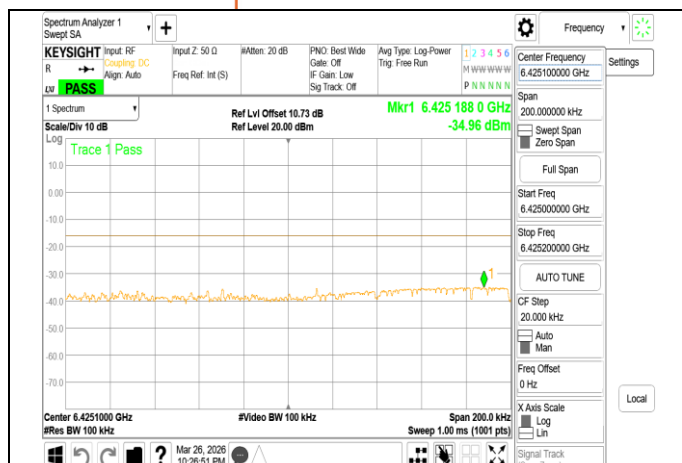
VLP 802.11be 80MHz Chain1 6385MHz Range2
