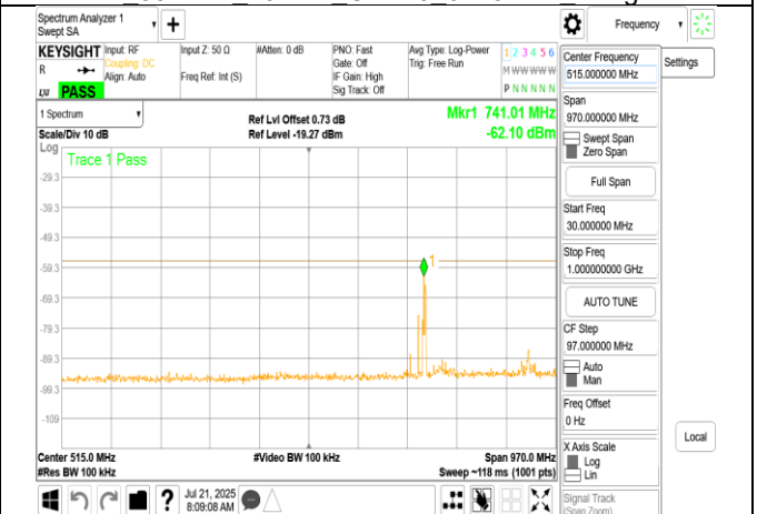
LPI 802.11a 20MHz Chain1 5955MHz Range1
