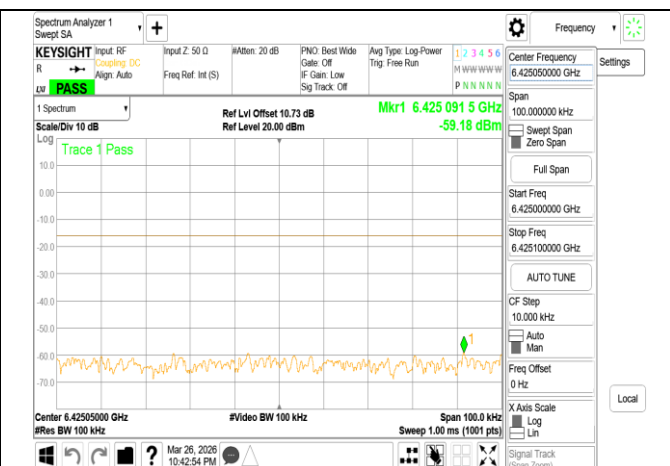
VLP 802.11be 160MHz Chain0 6185MHz Range2
