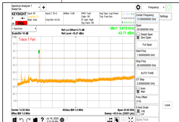
LPI 802.11n 40MHz Chain0 5965MHz Range2
