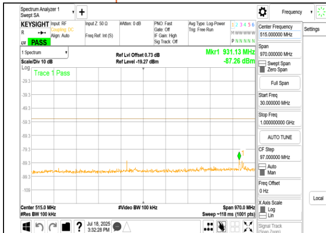
LPI 802.11ac 40MHz Chain0 5965MHz Range1
