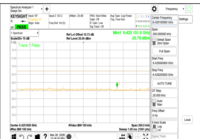
VLP 802.11be 80MHz Chain0 6385MHz Range2
