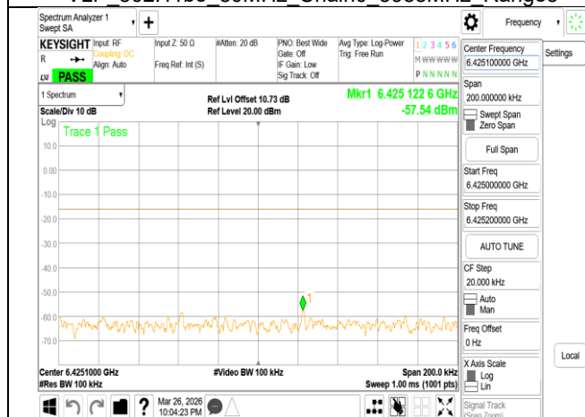
VLP 802.11be 80MHz Chain0 6145MHz Range2
