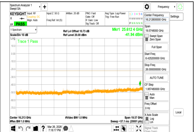
VLP 802.11ax 80MHz Chain1 5985MHz Range3
