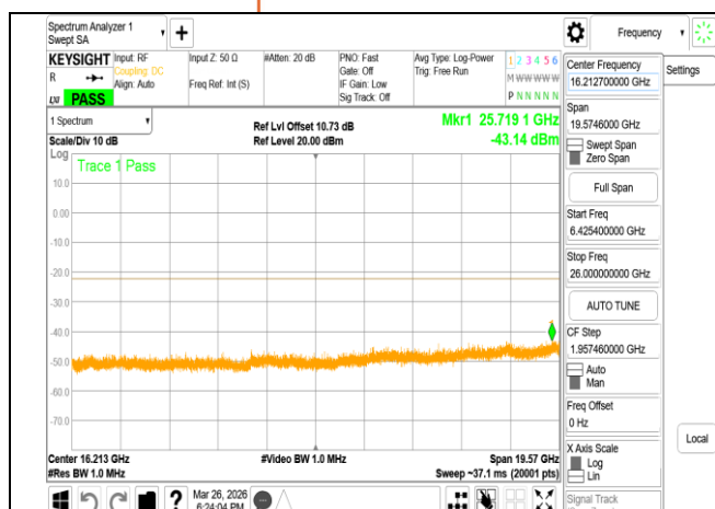
VLP 802.11ax 40MHz Chain0 5965MHz Range3
