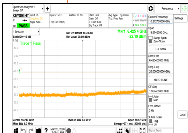
VLP 802.11ax 40MHz Chain0 6405MHz Range3
