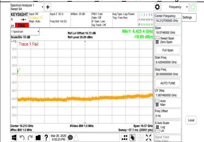
VLP 802.11be 40MHz Chain0 6405MHz Range3
