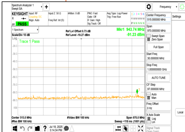
LPI 802.11a 20MHz Chain0 6415MHz Range1
