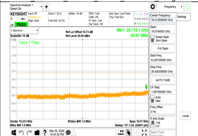
VLP 802.11be 160MHz Chain1 6185MHz Range3
