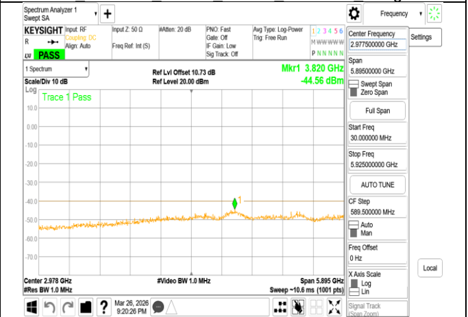
VLP 802.11be 40MHz Chain0 5965MHz Range1
