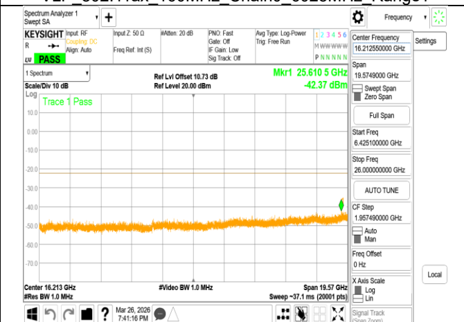
VLP 802.11ax 160MHz Chain0 6025MHz Range3
