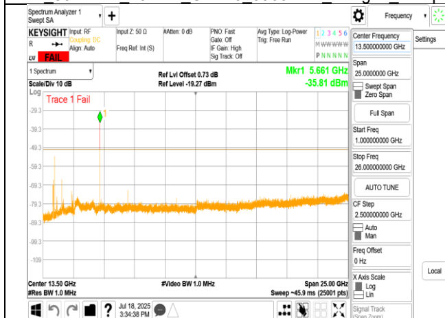
LPI 802.11ac 40MHz Chain0 6165MHz Range2
