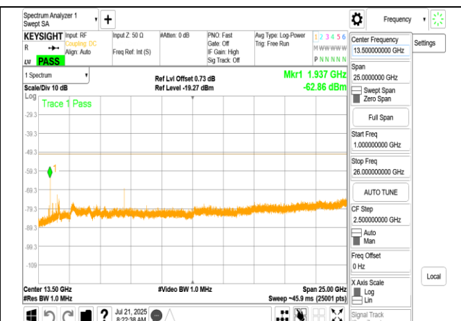
LPI 802.11n 40MHz Chain1 6165MHz Range2
