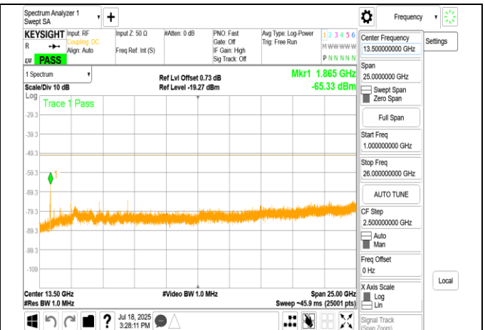
LPI 802.11ac 20MHz Chain0 5955MHz Range2
