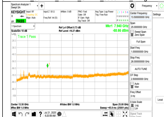
LPI 802.11n 40MHz Chain1 5965MHz Range2
