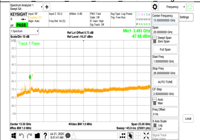
LPI 802.11ac 20MHz Chain1 6415MHz Range2
