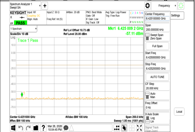
VLP 802.11be 80MHz Chain1 6145MHz Range2
