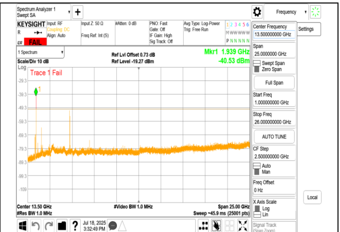
LPI 802.11ac 40MHz Chain0 5965MHz Range2
