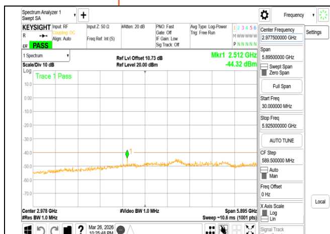
VLP 802.11be 80MHz Chain0 6385MHz Range1
