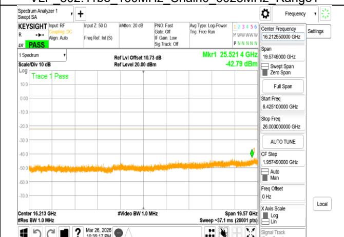
VLP 802.11be 160MHz Chain0 6025MHz Range3
