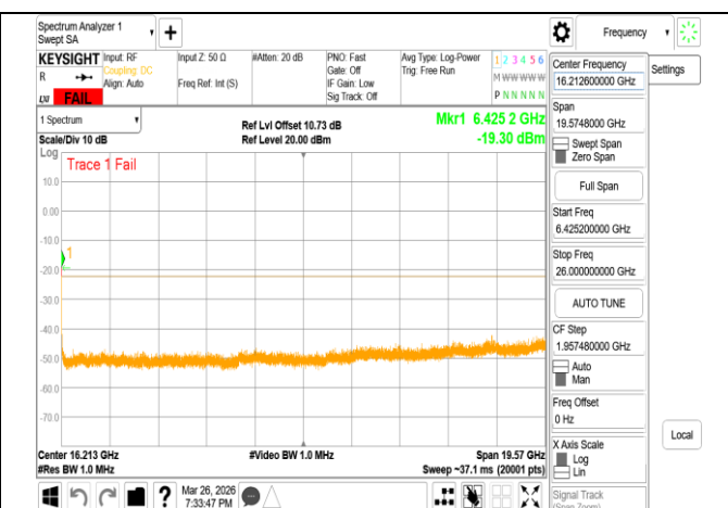
VLP 802.11ax 80MHz Chain1 6385MHz Range3
