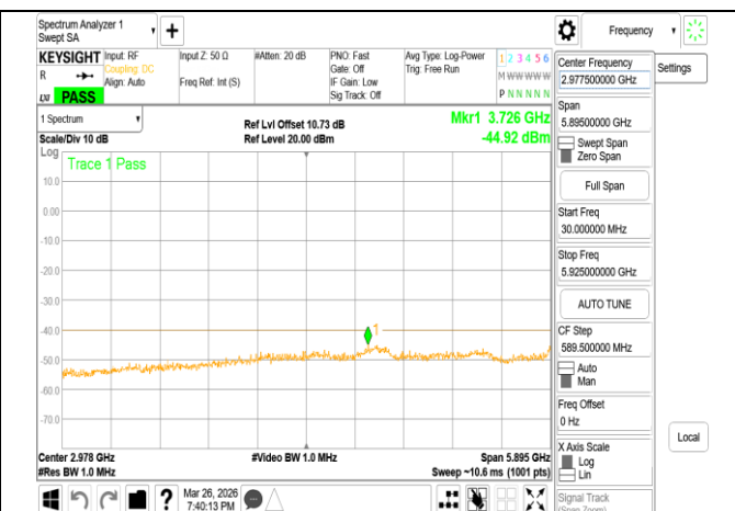
VLP_802.11ax_160MHz_Chain1_6025MHz_Range1
