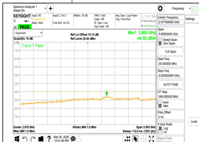
VLP 802.11be 160MHz Chain0 6185MHz Range1
