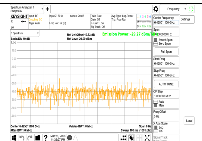
VLP_802.11be_320MHz_Chain0_6265MHz_Range2_Samp e
