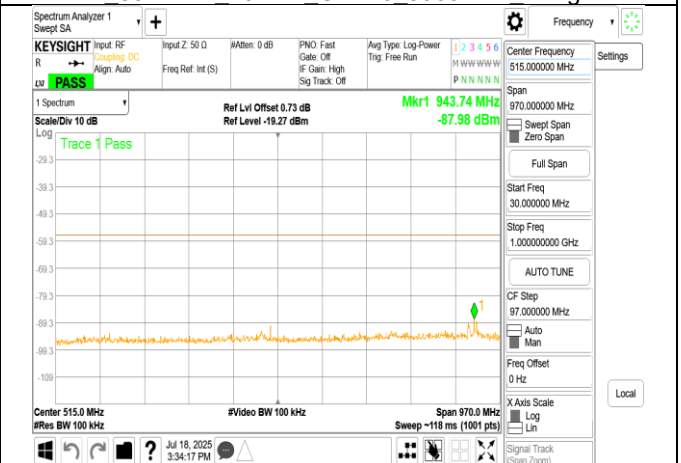
LPI 802.11ac 40MHz Chain0 6165MHz Range1
