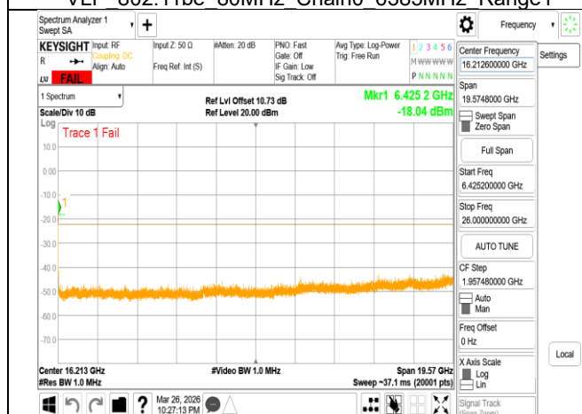
VLP 802.11be 80MHz Chain0 6385MHz Range3
