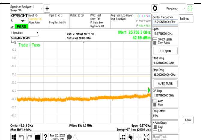
VLP_802.11ax_160MHz_Chain1_6025MHz_Range3
