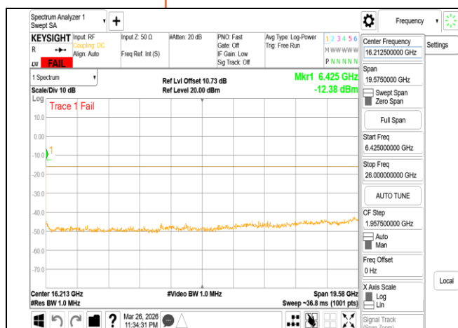
VLP_802.11be_320MHz_Chain0_6265MHz_Range2
