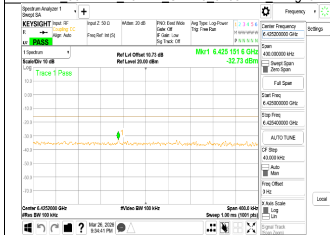
VLP 802.11be 40MHz Chain0 6405MHz Range2
