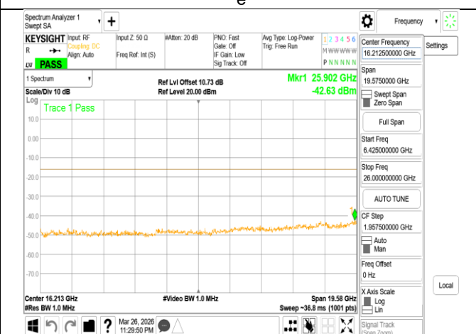
VLP_802.11be_320MHz_Chain1_6105MHz_Range2
