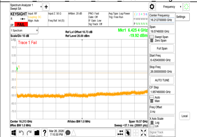
VLP 802.11ax 40MHz Chain1 6405MHz Range3
