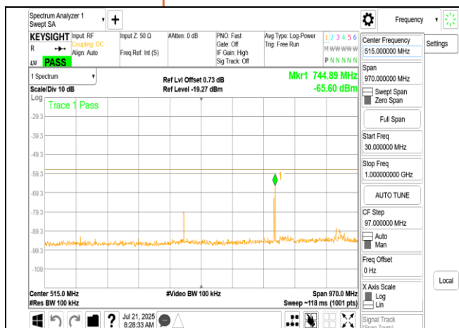
LPI 802.11ac 20MHz Chain1 6175MHz Range1
