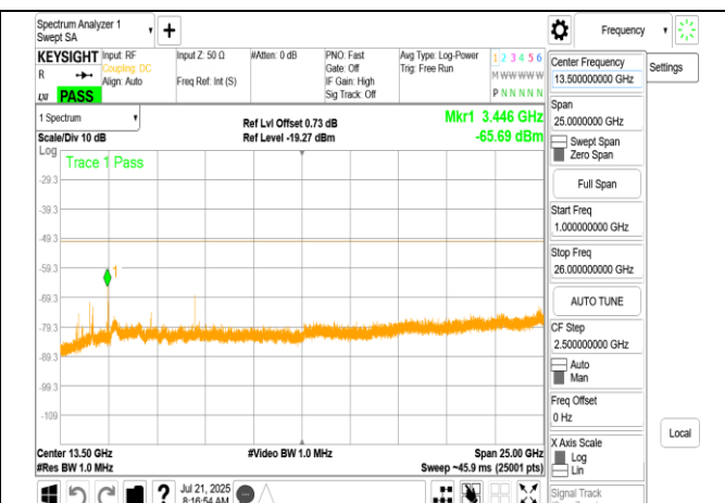
LPI 802.11n 20MHz Chain1 6175MHz Range2
