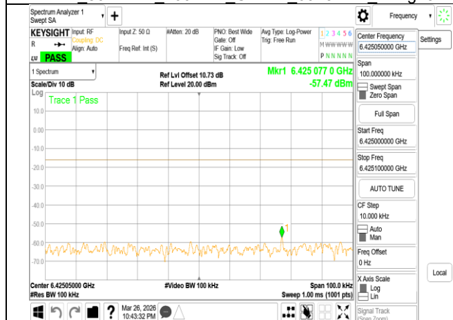
VLP 802.11be 160MHz Chain1 6185MHz Range2
