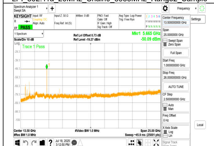
LPI 802.11a 20MHz Chain0 6175MHz Range2
