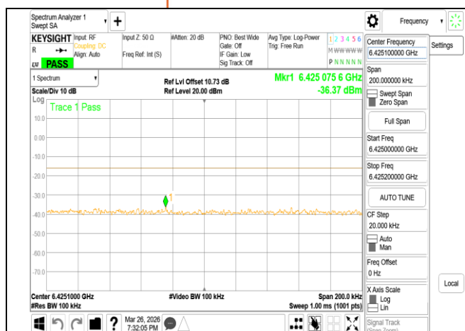
VLP 802.11ax 80MHz Chain1 6385MHz Range2
