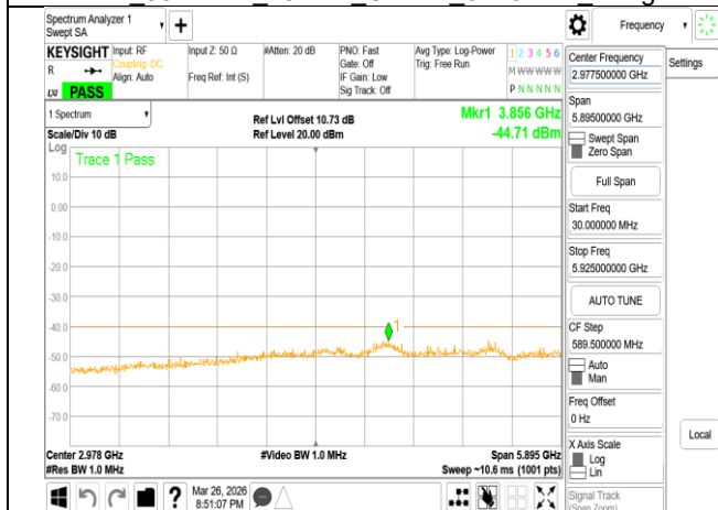
VLP 802.11be 20MHz Chain1 6415MHz Range1
