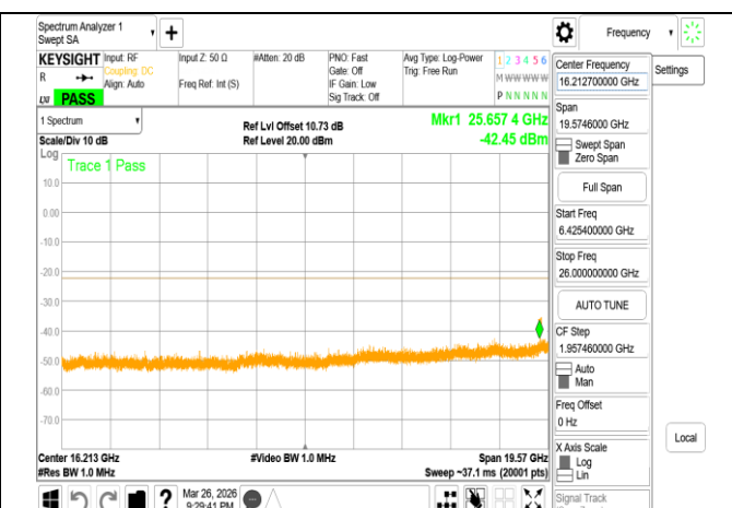
VLP 802.11be 40MHz Chain1 6165MHz Range3
