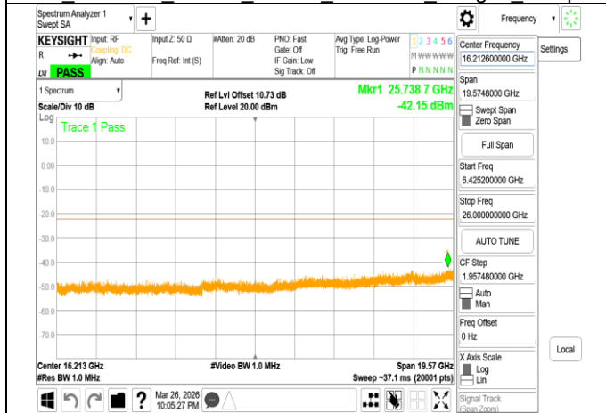
VLP 802.11be 80MHz Chain1 6145MHz Range3
