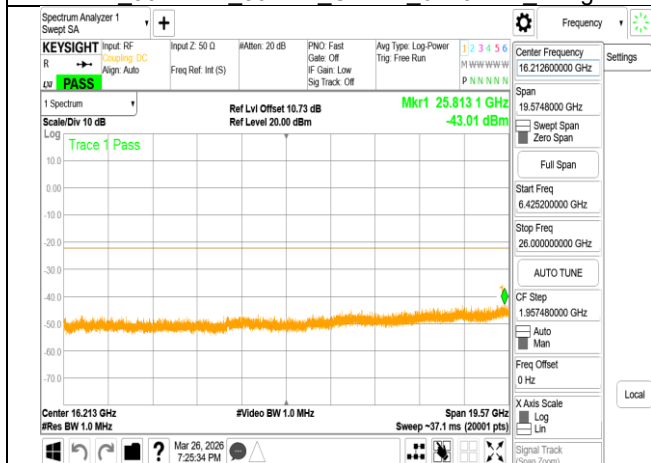
VLP 802.11ax 80MHz Chain1 6145MHz Range3
