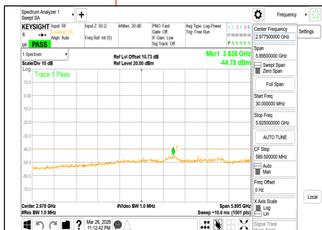
VLP 802.11be 160MHz Chain1 6345MHz Range1
