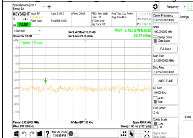
VLP 802.11ax 40MHz Chain1 6405MHz Range2
