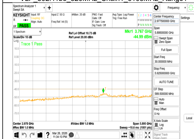
VLP_802.11be_320MHz_Chain1_6265MHz_Range1
