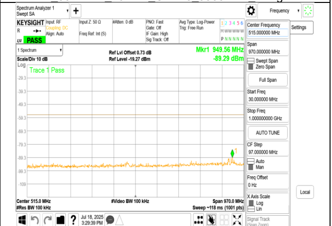
LPI 802.11ac 20MHz Chain0 6175MHz Range1
