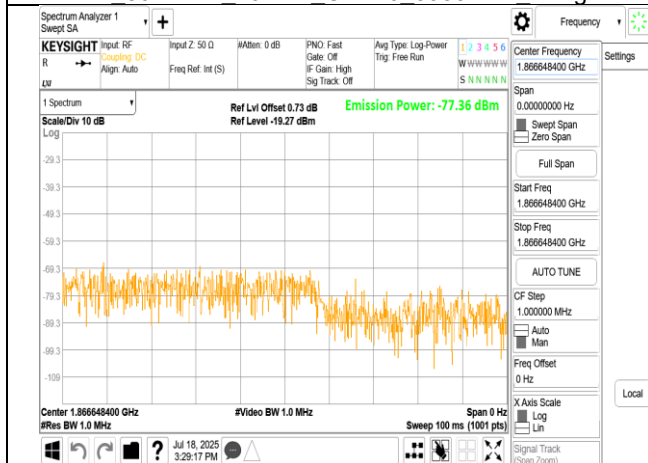
LPI 802.11ac 20MHz Chain0 5955MHz Range2 Sample
