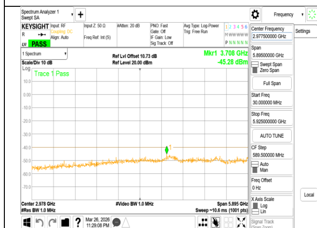
VLP_802.11be_320MHz_Chain1_6105MHz_Range1
