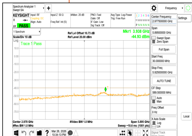
VLP 802.11be 160MHz Chain1 6025MHz Range1
