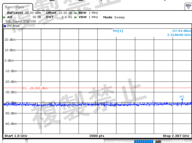
GFSK_Middle_DH1(1GHz~2.387GHz)
