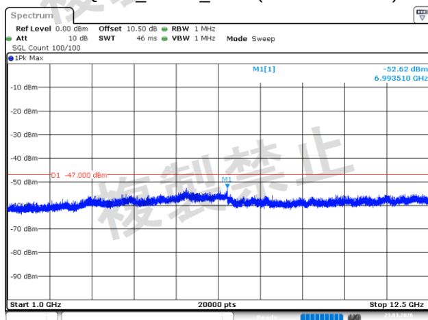
\pi/4 -DQPSK_Middle_2DH1(1GHz~12.5GHz)
