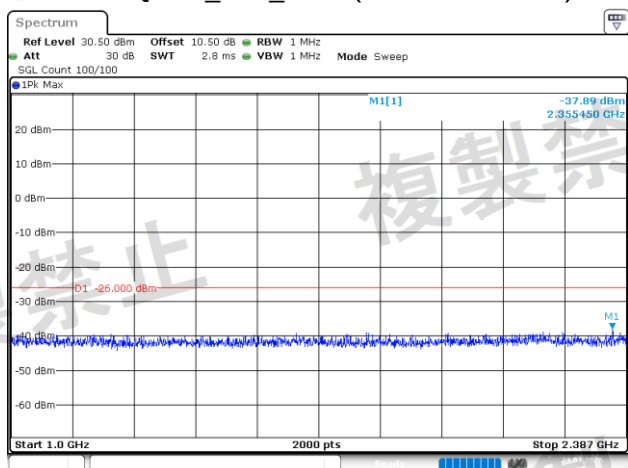
\pi/4 -DQPSK_Low_2DH1(1GHz~2.387GHz)
