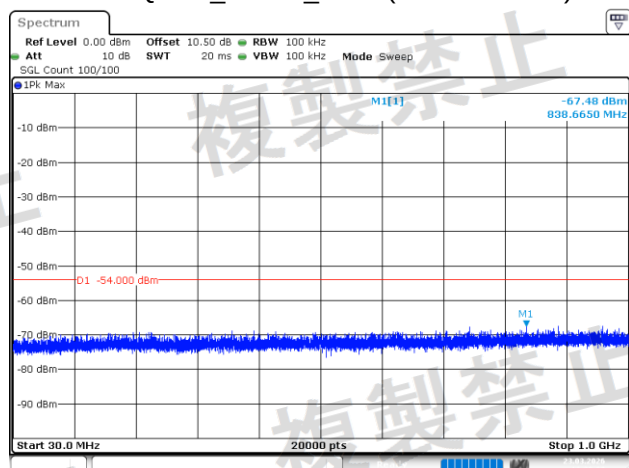
\pi/4 -DQPSK_Middle_2DH1(30MHz~1GHz)
