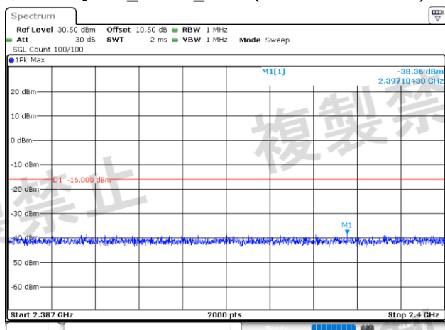
\pi/4 -DQPSK_Middle_2DH1(2.387GHz~2.4GHz)
