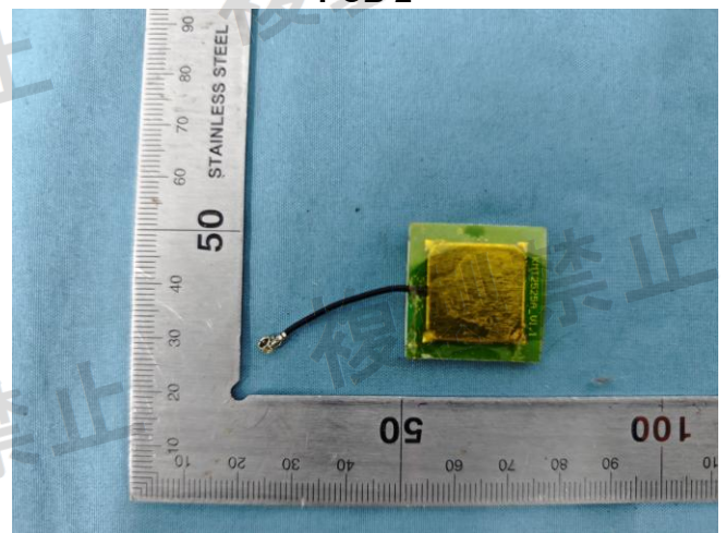
GPS Antenna
