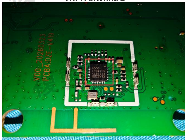
Bluetooth IC
