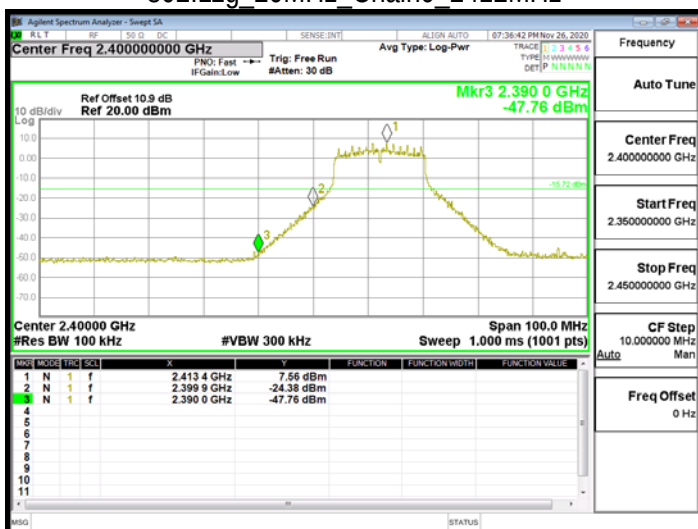
802.11g 20MHz Chain0 2412MHz
