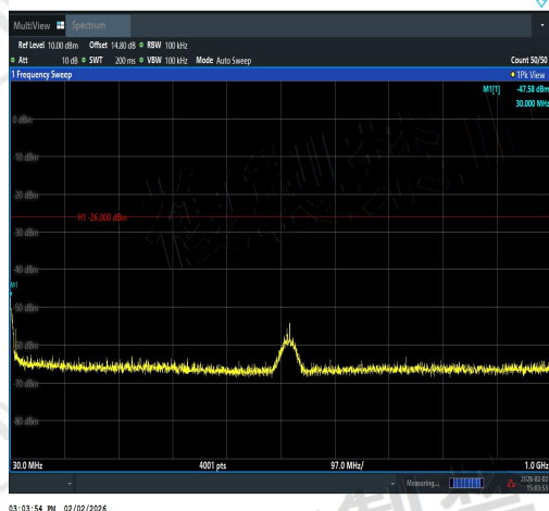
NTVN-11N40SISO-Ant1-2462-30~1000-PASS
