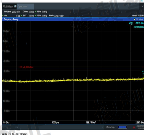
NTVN-11N40SISO-Ant2-2462-1000~2387-PASS
