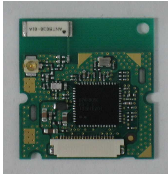
Top View2 *1
