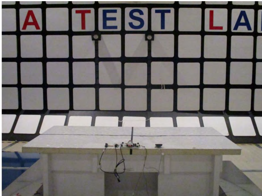
Mode 1_1 GHz 以下 背面
