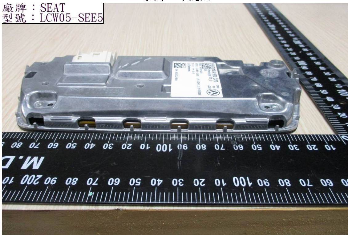
系列 2 外觀照
