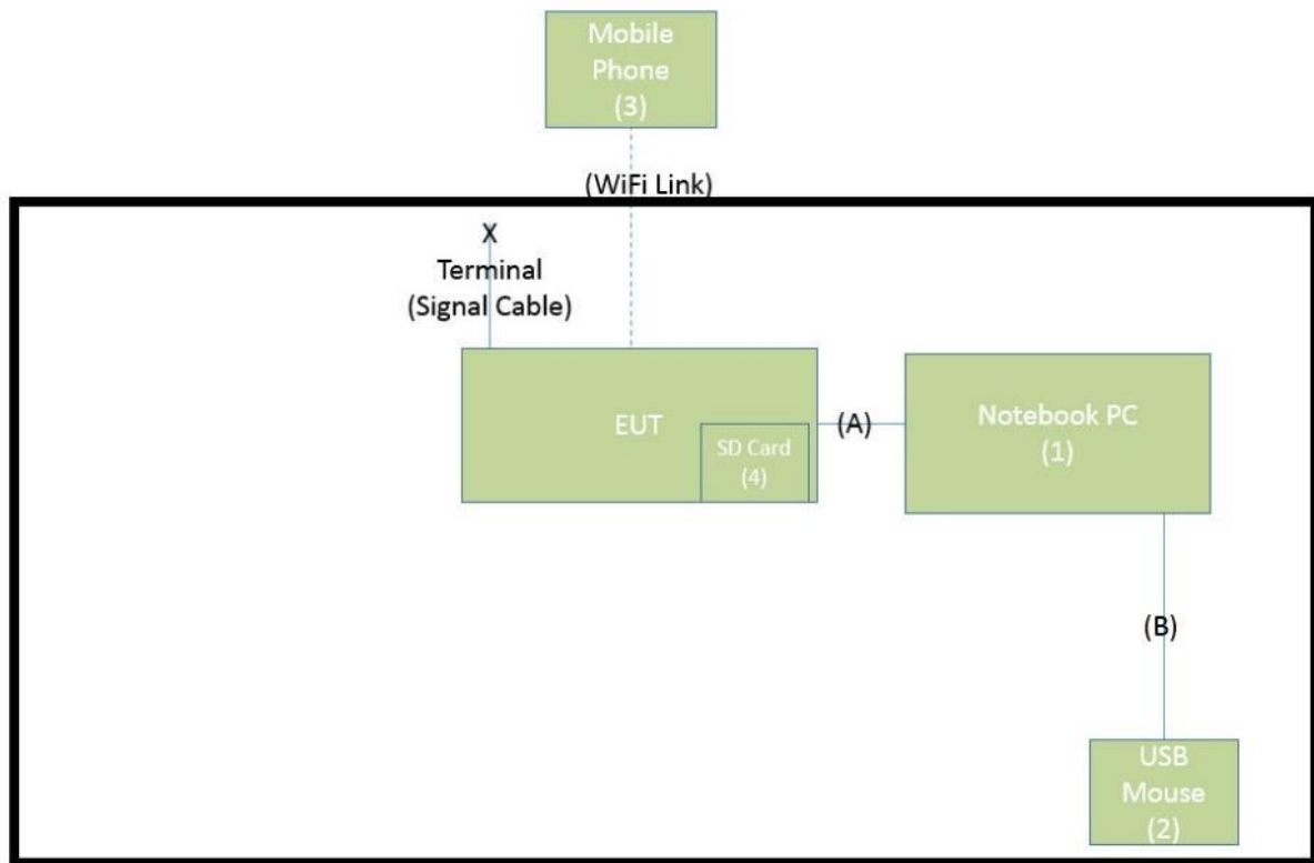
待測物測試配置圖 (Mode5)
