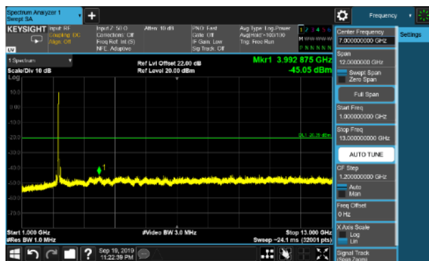
802.11 g CH06 (2437MHz)
