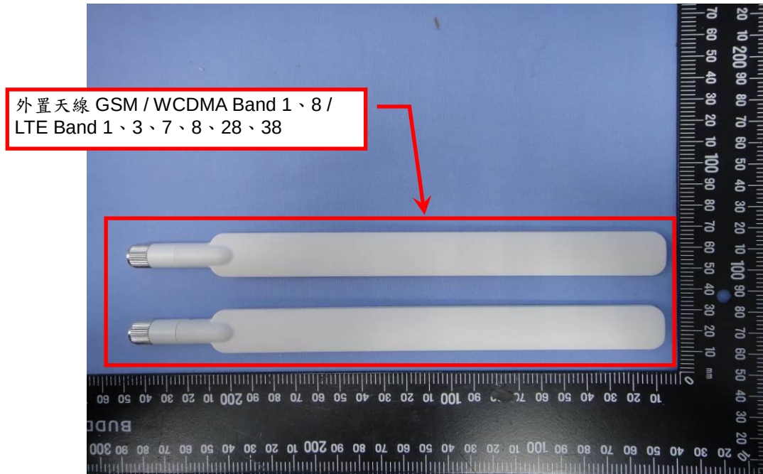
EUT Photo (16)
