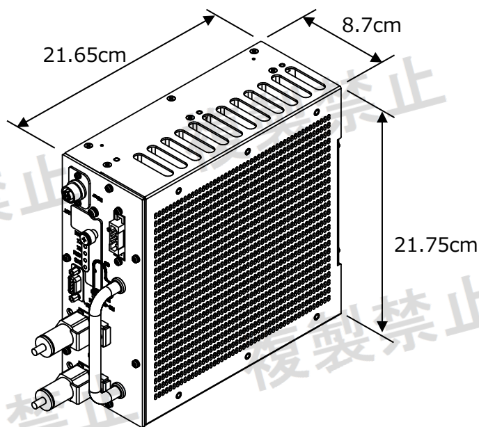
MS-BBU 外觀圖
