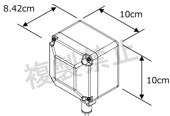
MS-RFU-W 外觀圖
