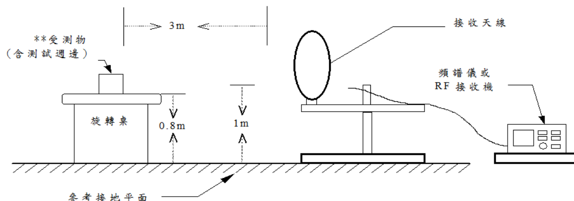
圖 1:量測頻率9kHz ~ 30MHz之測試配置
