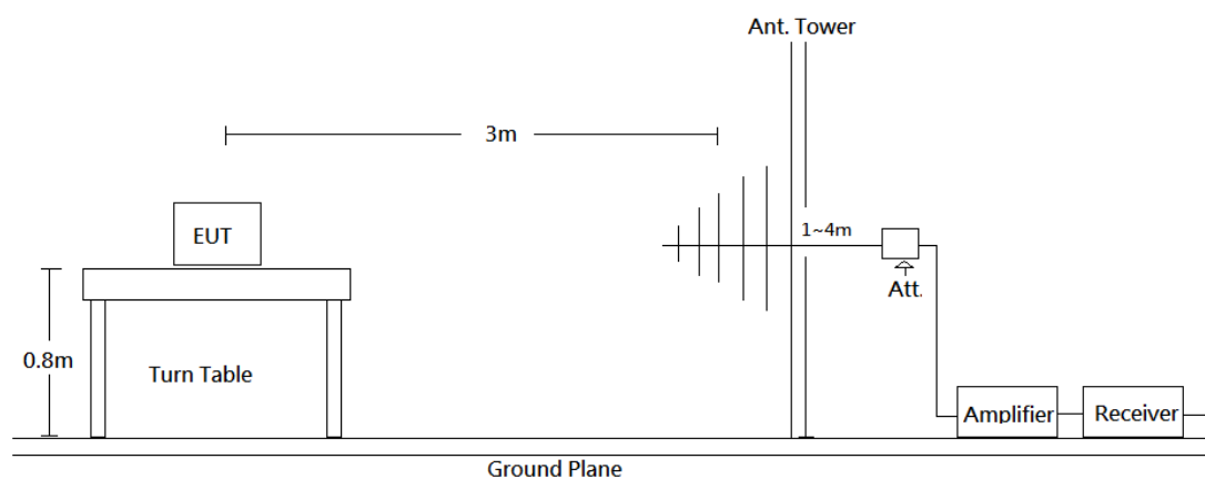
圖 2:量測頻率30MHz~1GHz之測試配置
