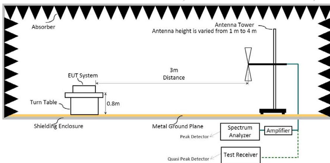
圖 2: 量測頻率高於 1GHz 之測試配置 (No.1 3m Semi Anechoic Chamber)
