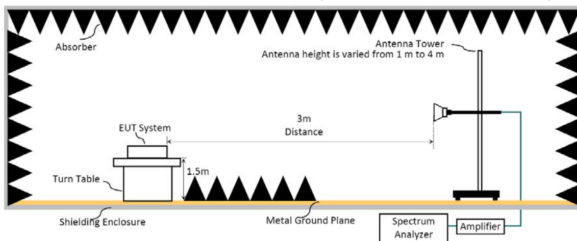
圖 2: 量測頻率高於 1GHz 之測試配置 (No.1 3m Semi Anechoic Chamber)
