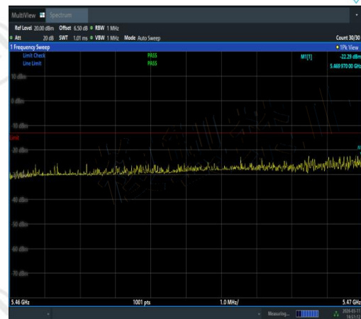
NTVN-11N40SISO-Ant1-5510-5460~5470-PASS
