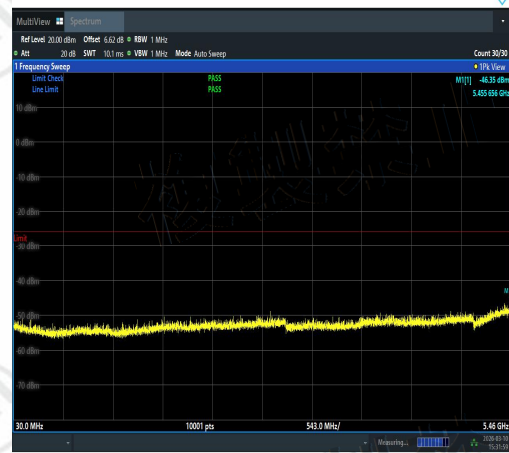
NTVN-11AC20SISO-Ant2-5700-30~5460-PASS
