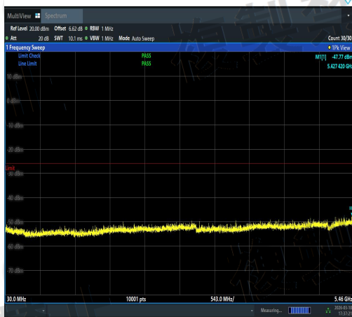
NTVN-11AC20SISO-Ant3-5700-30~5460-PASS
