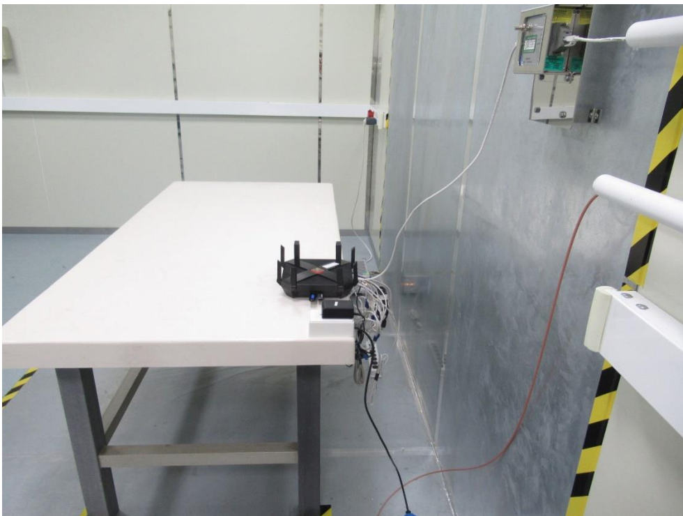
電源傳導測試 側面照 - 0.15MHz ~ 30MHz (Normal Mode)
