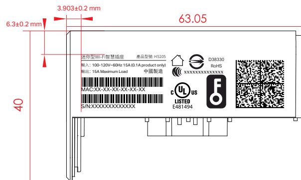
尺寸图
